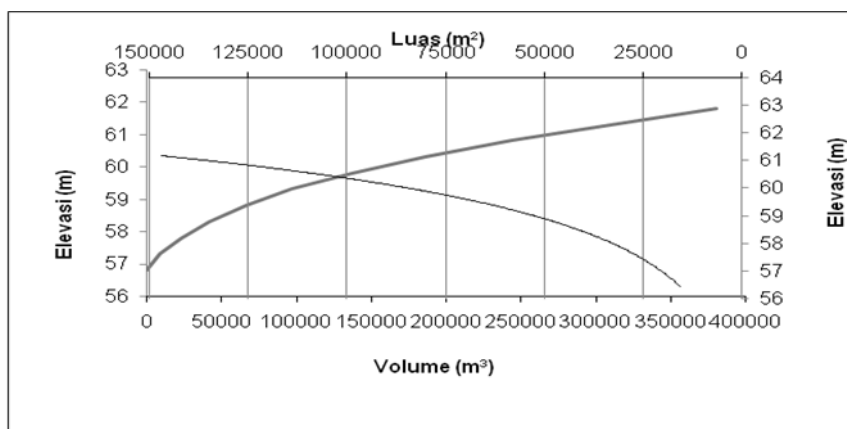
Gambar 4. Kurva Tampungan Embung Alternatif II
