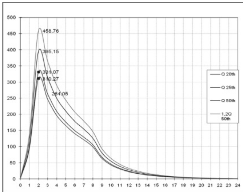
Gambar 5. 15 Hidrograf Debit di DAS Pamekasan
