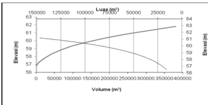
Gambar 4. [0] Kurva Tampungan Embung Alternatif II
