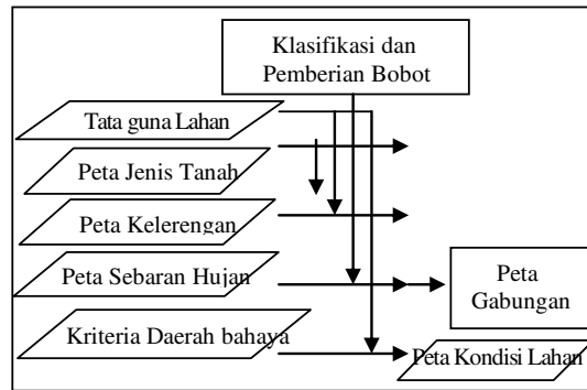
Gambar 1. Alir Proses Identifikasi Kondisi Lahan
