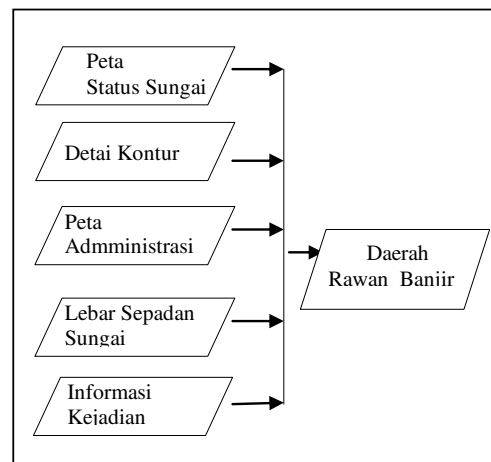
Gambar 3. Proses Analisa Daerah Rawan Banjir
