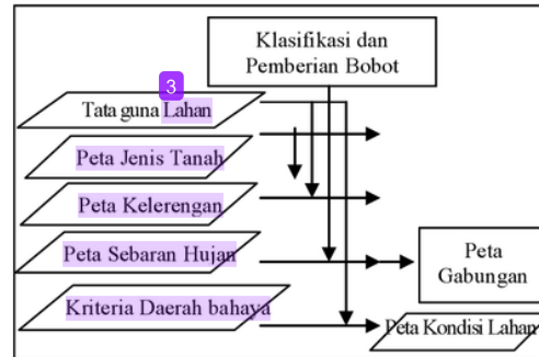
Gambar 1. Alir Proses Identifikasi Kondisi Lahan
