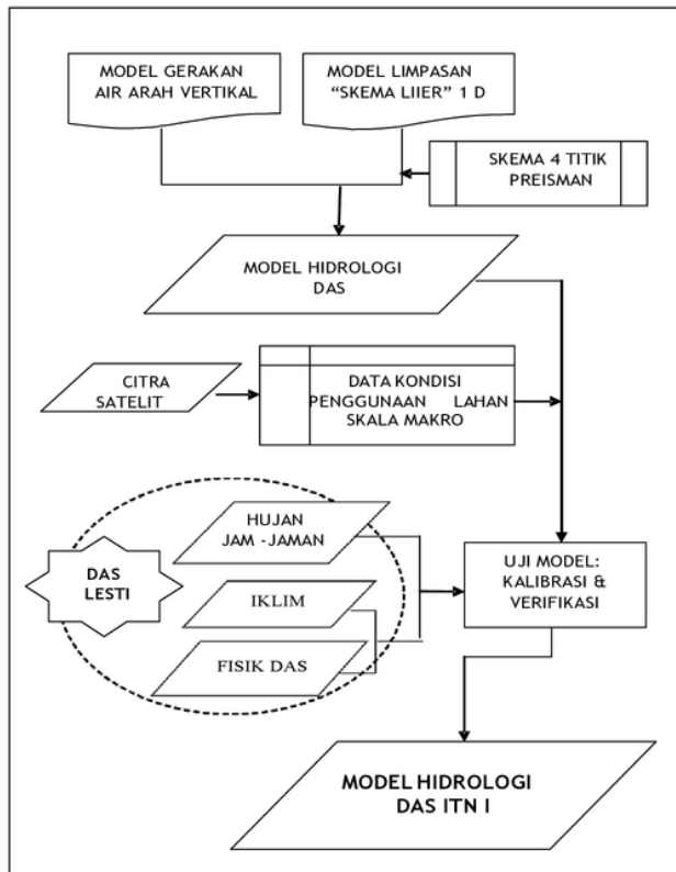
Gambar 2 Skema Pemodelan
