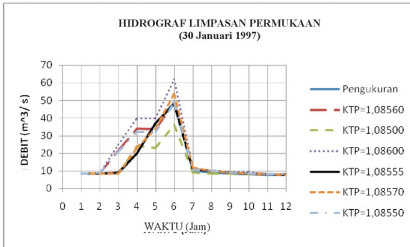
Gambar 4 Hidrograf Debit Banjir dengan Berbagai Nilai KTP
