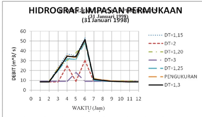
Gambar 3 Hidrograf Debit Banjir Dengan Berbagai Nilai DT
