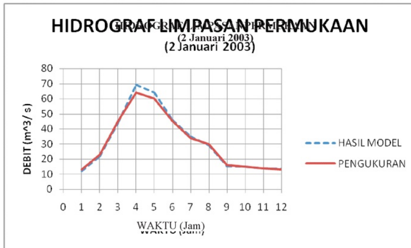
Gambar 5 Hidrograf Debit Dalam Verifikasi KTP dan DT
