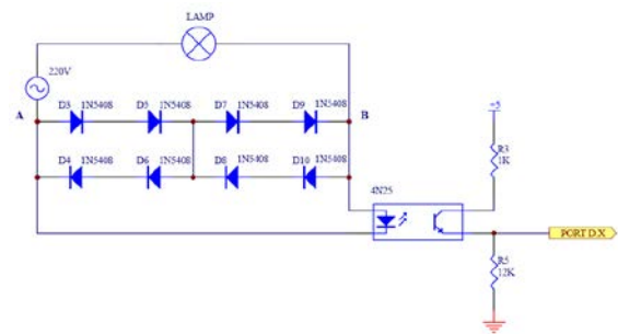
Gambar 4. Rangkaian Detektor Arus.
