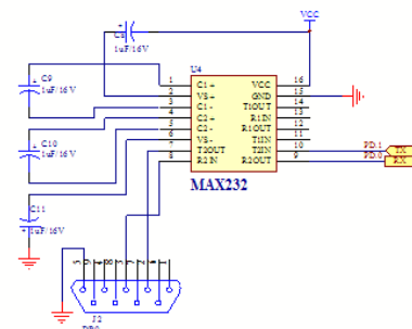
Gambar 6. Rangkaian RS232 menggunakan IC MAX232.
