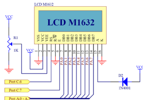
Gambar 7. Rangkaian LCD.
