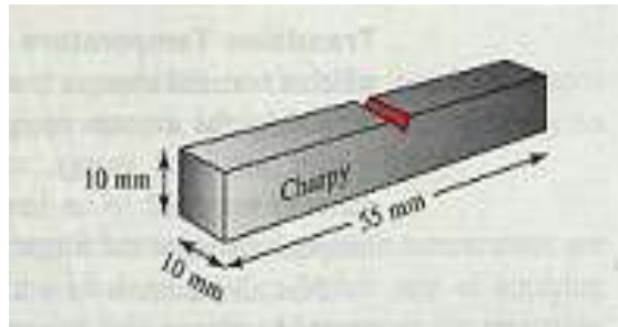
Gambar 5. spesimen benda uji impact
