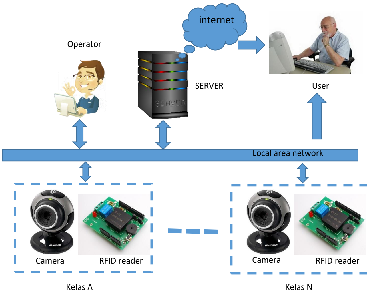
Gambar 2. Blok diagram ruang kelas pintar
