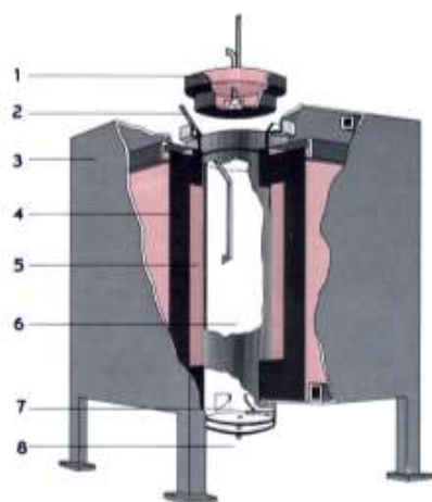
Gambar 1. Konstruksi dapur fluidised bed [Reynoldson, 2003]
