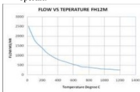
Gambar 3. Grafik Temperatur terhadap aliran gas pada operasi fluidised bed furnace
