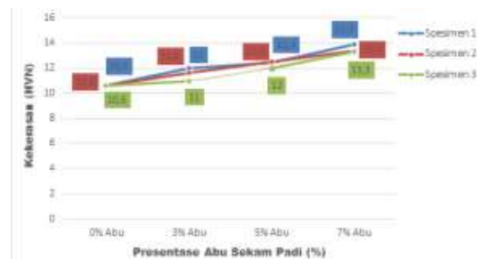
Gambar 6. Perbandingan Fraksi Volume Abu Sekam Padi dan HVN
