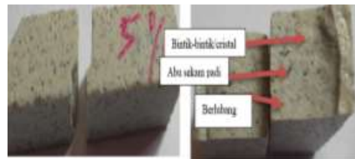
Gambar 9. Foto Makro 95% Plasktik : 5% Abu Sekam Padi
