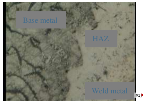
Gambar 24 Struktur mikro pada base metal, haz, dan weld metal (Perbesaran 400x)
