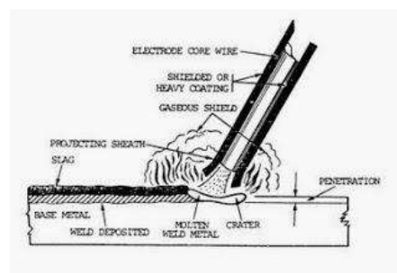
Gambar 1 Las Busur dengan Elektroda Terbungkus
