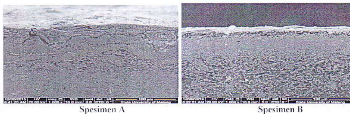
Gambar 3. Struktur mikro SEM EDAX (Pemb. 1000 x)
