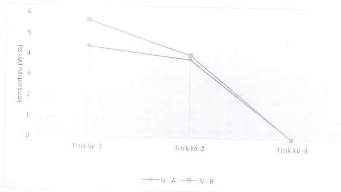
Gambar 4. Grafik Perbandingan Kadar N Spesimen A dan B
