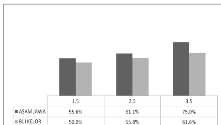
Grafik 7. Efisiensi pemisahan TSS pada 40 rpm.
