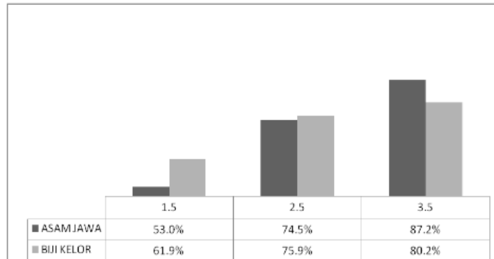
Grafik 2. Efisiensi Pemisahan COD pada 40 rpm.
