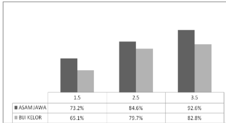
Grafik 1. Efisiensi Pemisahan COD pada 20 rpm.
