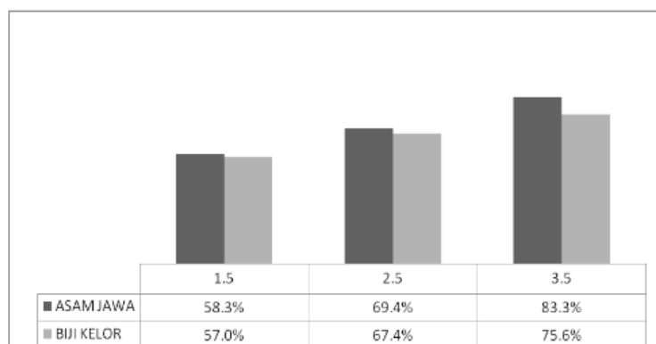
Grafik 6. Efisiensi Pemisahan TSS pada 20 rpm.
