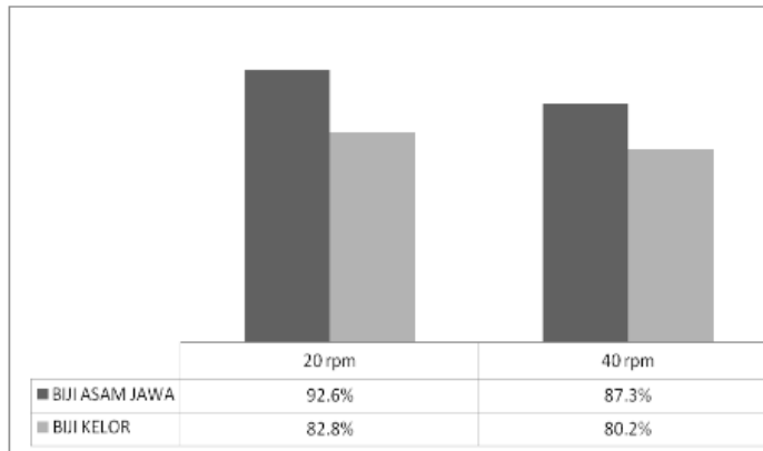
Grafik 5. Efisiensi Pemisahan COD dengan dosis biokogulan 2,5 gr/l.
