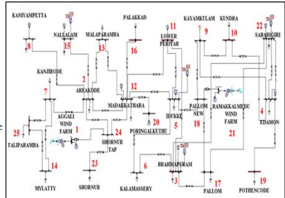
Fig. 2. Kerala grid 220kV 25-bus system
