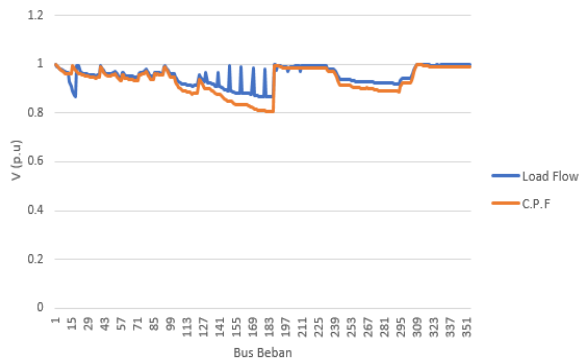
Gambar 12. Grafik Profil Tegangan pada Sistem Maumere pada Saat CPF (Continuation Power Flow) pada Case 2.
