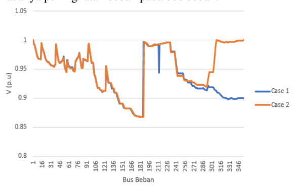
Gambar 13. Grafik Profil Tegangan Pada Sistem Maumere Pada Saat Load Flow Pada Case 1 dan Case 2.
