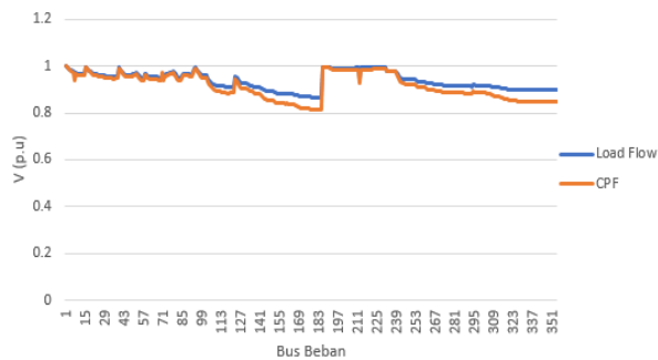
Gambar 8. Grafik Profil Tegangan pada Sistem Maumere Load Flow dan CPF (Continuation Power Flow) pada Case 1
