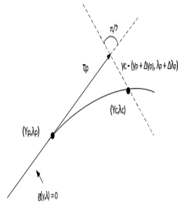
Gambar 3. Continuation Power Flow: Corrector Step Diperoleh Melalui Persimpangan Tegak Lurus. [7]
