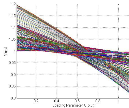
Gambar 5. Kurva Untuk Semua Tegangan Bus Beban Pada Case 1
