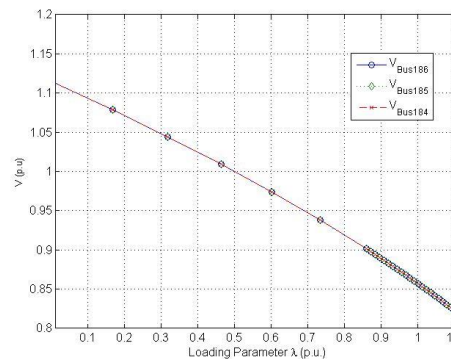
Gambar 6. Kurva Untuk Tiga Tegangan Bus Beban Terlemah Pada Case 1.
