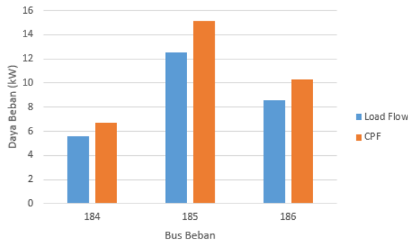
Gambar 7. Grafik Beban Kondisi Base Case
