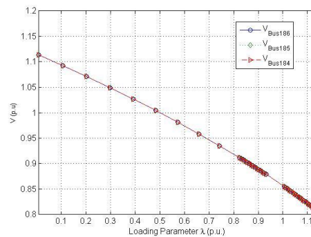
Gambar 10. Kurva untuk Tiga Tegangan Bus Beban Terlemah pada Case 2.
