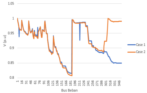
Gambar 16. Grafik Profil Tegangan Pada Sistem Maumere Pada Saat Continuation Power Flow Pada Case 1 dan Case 2
