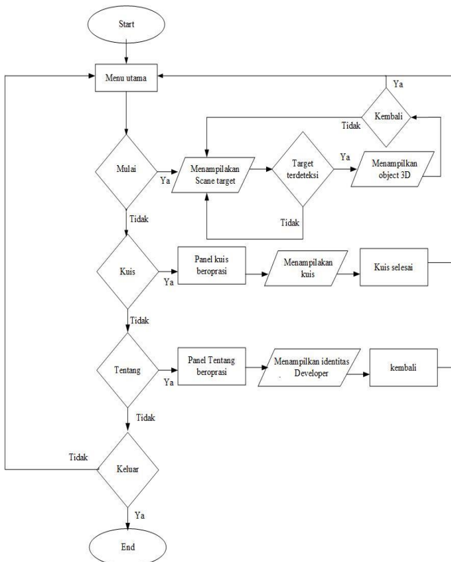
Gambar 3.3 Flowchart Aplikasi
