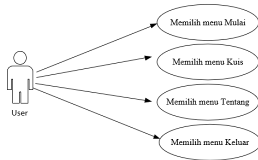
Gambar 3.4 UseCase Aplikasi
