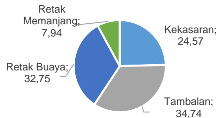
Gambar 4 Diagram Prosentase Kerusakan Jl. Joyo Utomo
