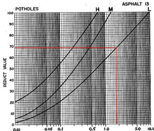
Gambar 6 Kurva Deduct Value Untuk Kerusakan Lubang
