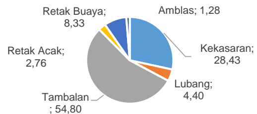
Gambar 5 Diagram Prosentase Kerusakan Jl. Joyo Tambaksari
