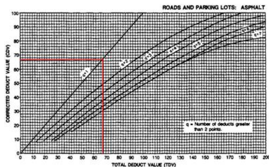
Gambar 7 Kurva Hubungan TDV dan nilai CDV Jl. Joyo Agung STA 0+000 sd 0+100
