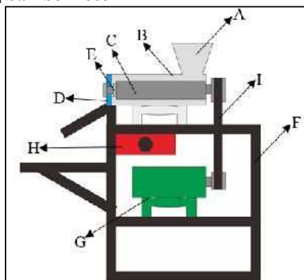
Gambar 1. desain penggiling sambel pecel
