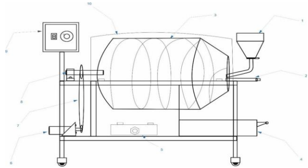
Gambar 2. Mesin pengarangan
