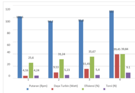
Grafik 5. Hubungan Jumlah Blade Terhadap Putaran, Torsi, Daya Turbin dan Efisiensi
