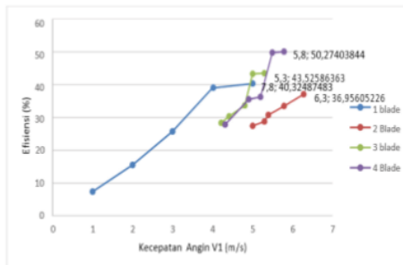
Grafik 3 Hubungan kecepatan angin (m/s) dan Efisiensi (%)
