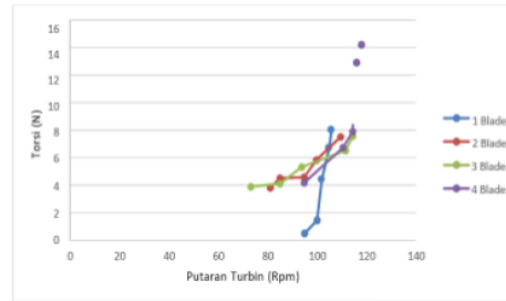
Grafik 4 Hubungan putaran turbin (rpm) dan torsi (N)
