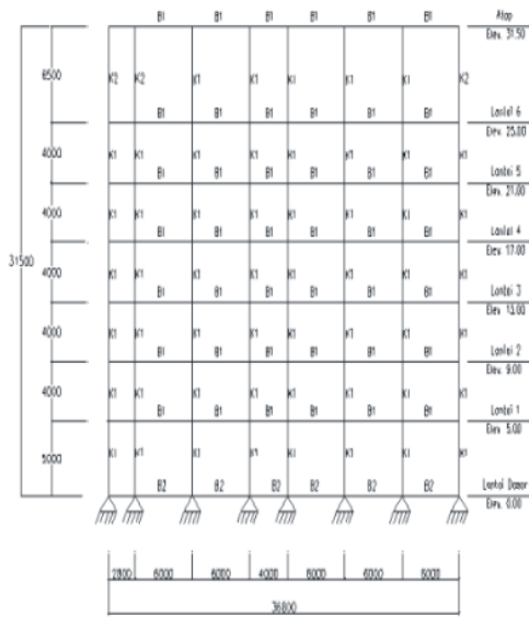
Gambar 3. Gambaran Umum Gedung (Memanjang)
