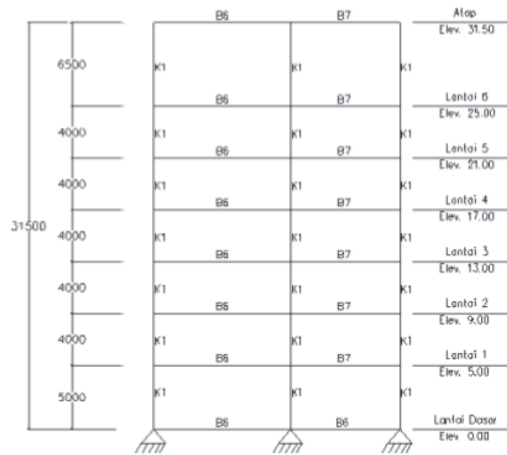
Gambar 4. Gambaran Umum Gedung (Melintang)
