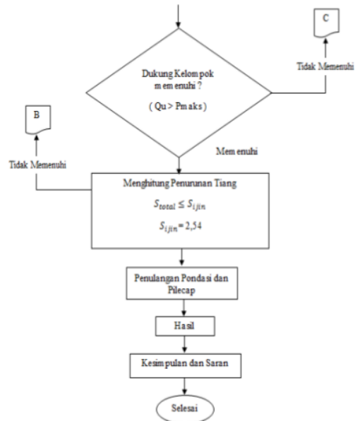
Gambar 5. Bagan Alir Perencanaan
