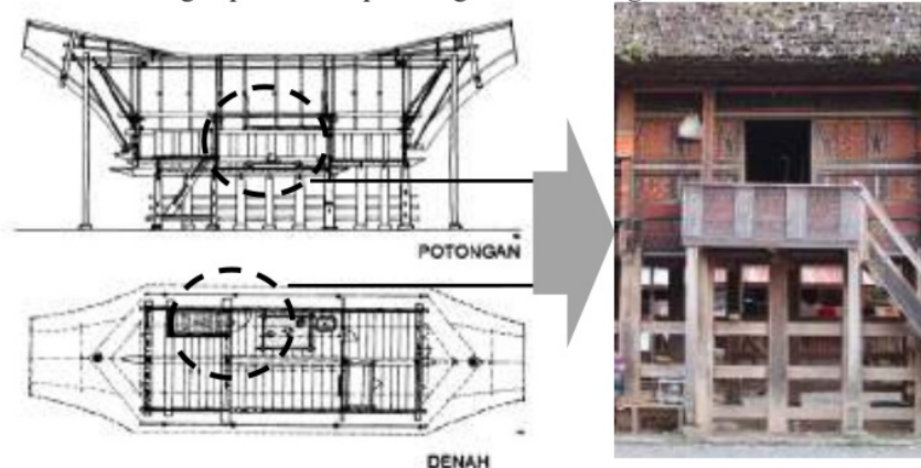
Gambar 4. 38 Pintu Tongkonan yang dipasang pada bagian timur
