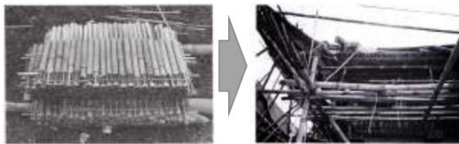
Gambar 4. 35 Proses Massu'duk penggantian atap Tongkonan
