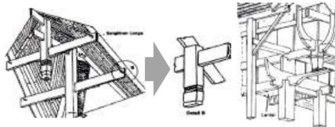
Gambar 4. 34 Proses Mang'lo'po pelubangan kayu
