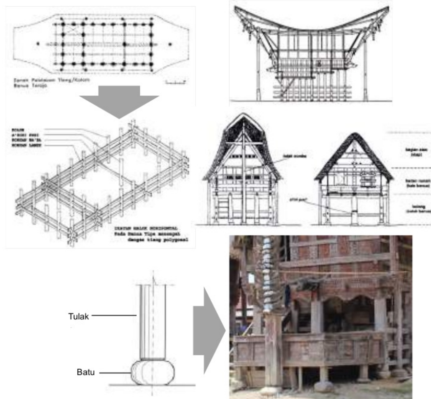
Gambar 4. 39 Struktur tiang – tiang pondasi Tongkonan
