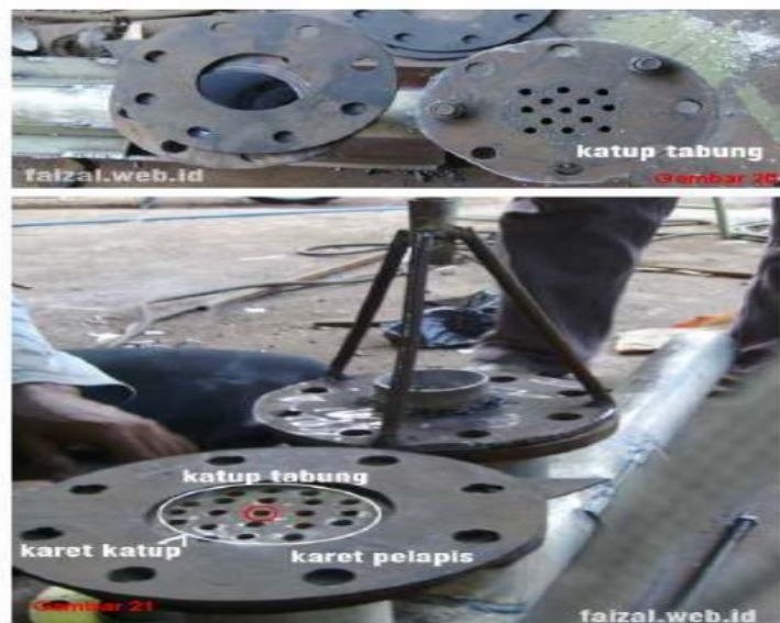
Gambar 20-21: Katup tabung pompa hidram.
