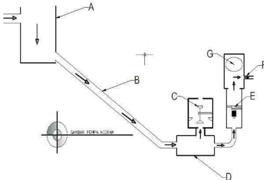
Gambar 4.1. Skema Pompa Hidram
