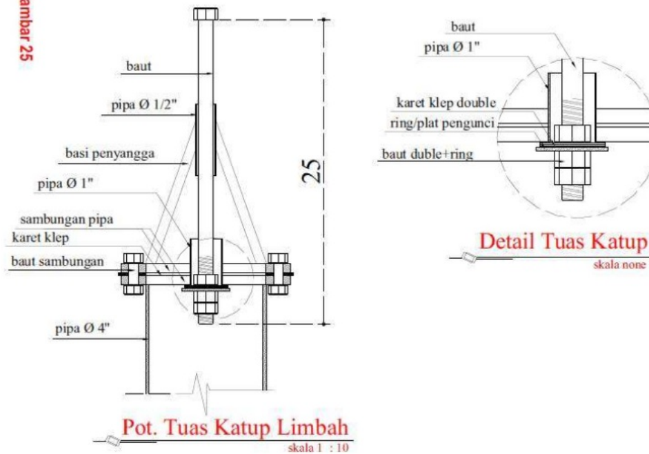
Gambar 25: Skema Katup Limbah dan Tuasnya
