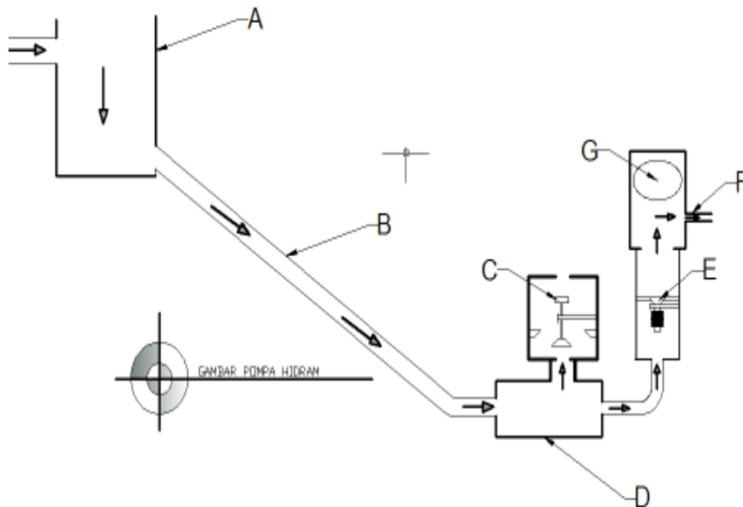
Gambar 2.5 Skema Penelitian Pompa Hidram
