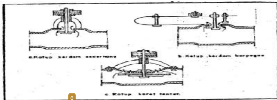
6 Gambar 2.2. Contoh Desain Katup Limbah
