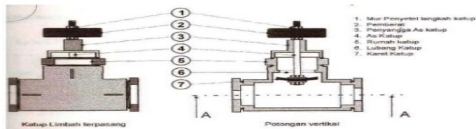
Gambar 2.3 Komponen katup buang jenis kerdam
