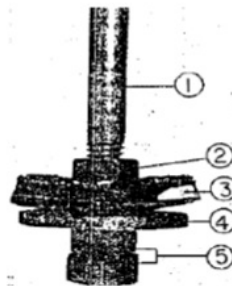
Gambar 2.4 Bagian – Bagian Katup Buang.
