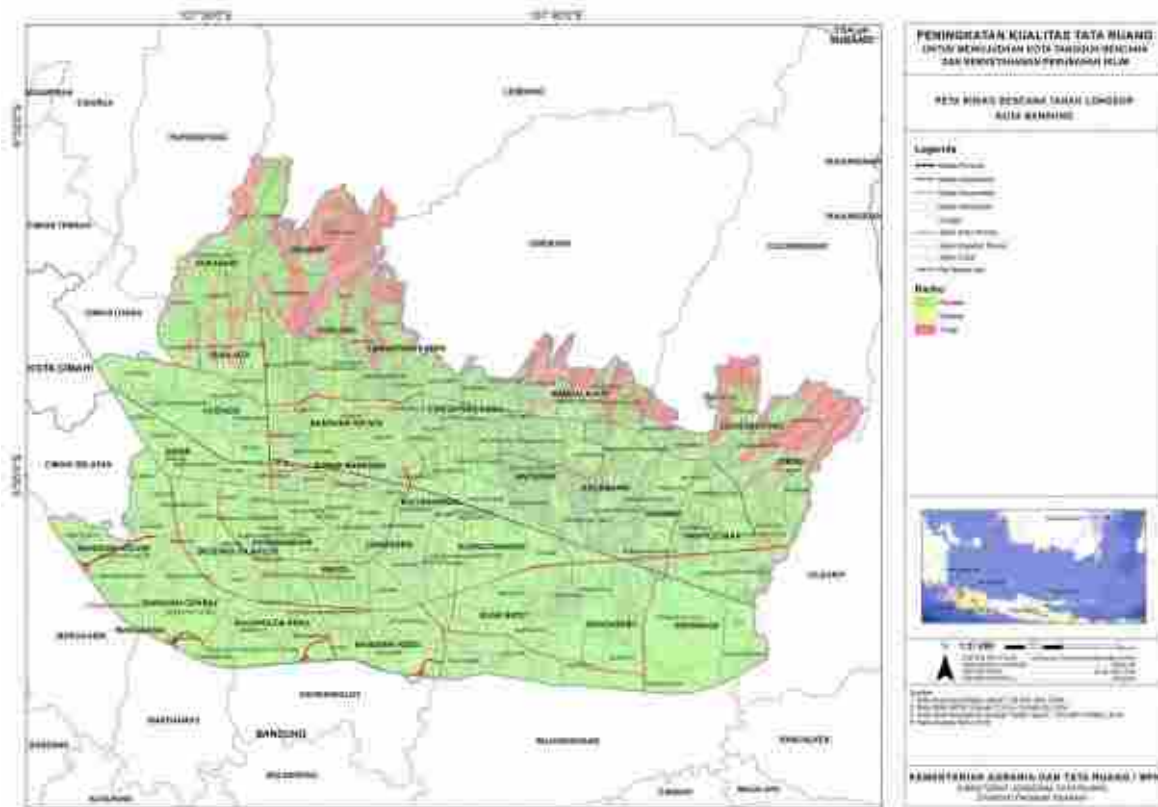
Gambar 21 Peta Tingkat Risiko Longsor Kota Bandung
