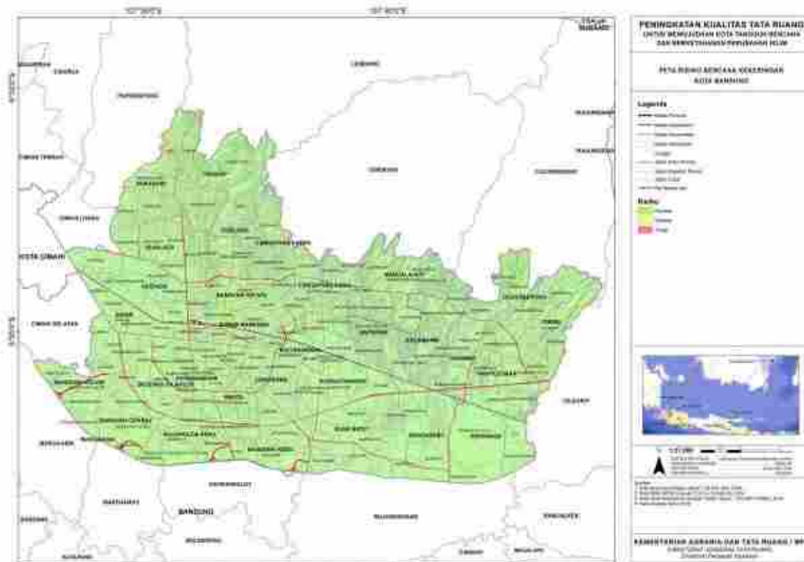
Gambar 22 Peta Tingkat Risiko Kekeringan Kota Bandung
