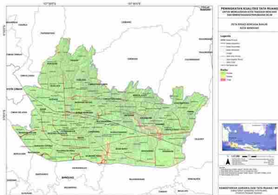
Gambar 20 Peta Tingkat Risiko Banjir Kota Bandung
