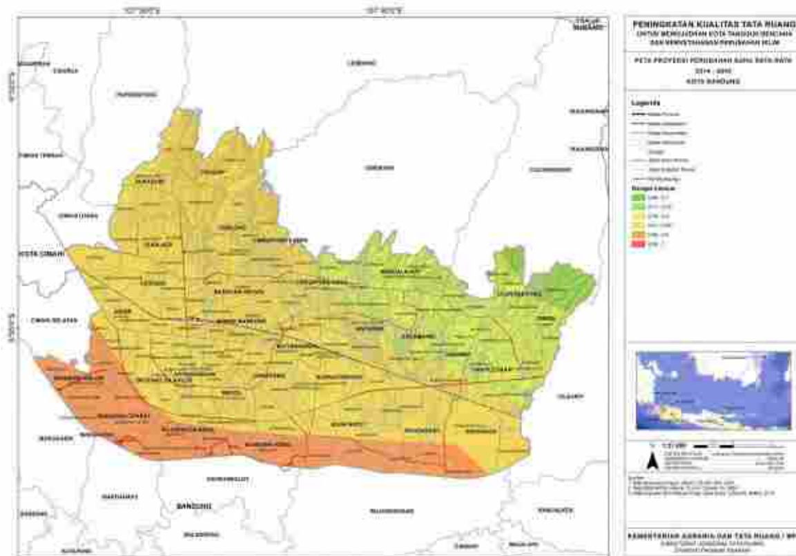
Gambar 26 Peta Proyeksi Suhu
