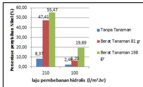
Grafik 4 Hubungan Persentase Penyisihan Nikel (%) terhadap laju pembebanan hidrolis dengan reaktor menggunakan Tanaman Lotus dan tanpa tanaman
