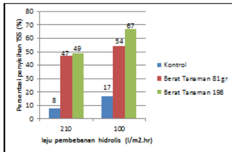
Grafik 1. Hubungan Persentase Penyisihan TSS (%) terhadap laju pembebanan hidrolis dengan reaktor menggunakan Tanaman Bambu Air dan tanpa tanaman
