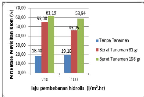
Grafik 6 Hubungan persentase penyisihan Total krom (%) terhadap dengan reaktor menggunakan Tanaman Lotus dan tanpa tanaman
