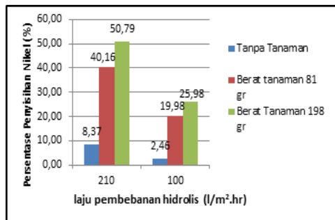
Grafik 3 Hubungan Persentase Penyisihan Nikel (%) terhadap laju pembebanan hidrolis dengan reaktor menggunakan Tanaman Bambu Air dan tanpa tanaman.
