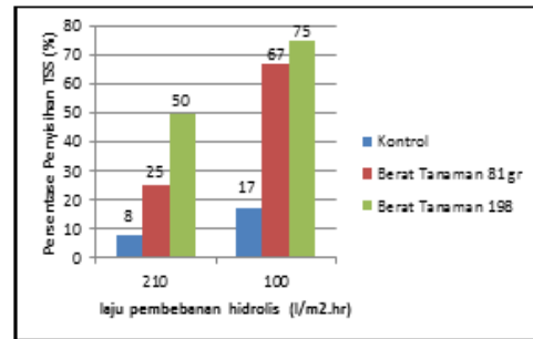
Grafik 2. Hubungan Persentase Penyisihan TSS (%) terhadap laju pembebanan hidrolis dengan reaktor menggunakan Tanaman Lotus dan tanpa tanaman.
