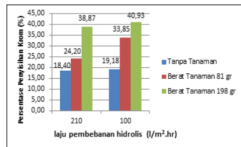
Grafik 5 Hubungan persentase penyisihan Total krom (%) terhadap dengan reaktor menggunakan Tanaman Bambu Air dan tanpa tanaman
