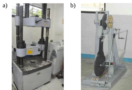
Gambar 4. a) Mesin Uji Tarik dan b) Mesin Uji Impact
