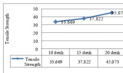
Grafik 1. Hubungan Tensile Strength Terhadap Waktu Penekanan
