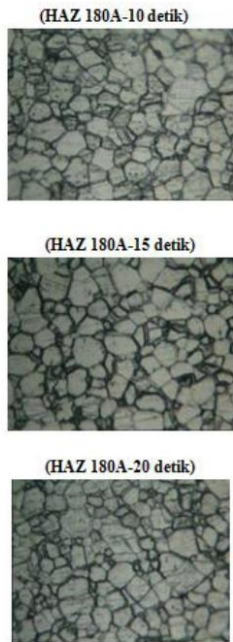
Gambar 8. Hasil foto mikro daerah HAZ waktu tekan (10,15,20 detik)
