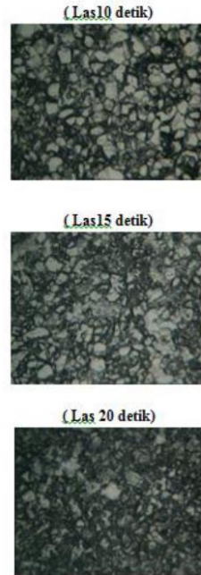
Gambar 9. Daerah las waktu penekanan (10, 15, 20 detik) perbesaran 400x
