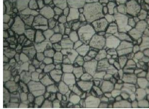
Gambar 7. Hasil foto mikro logam induk perbesaran 400X
