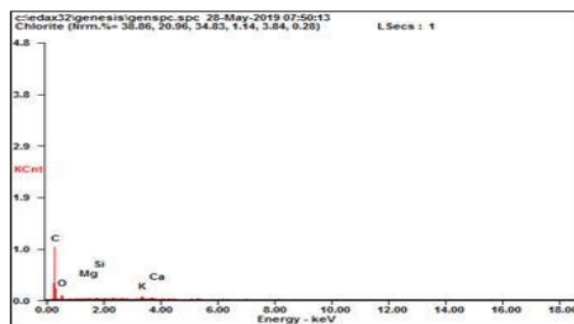
Gambar 1. Grafik kandungan unsur kimia dari partikel arang sampah organik.
