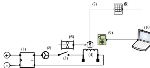
Gambar 2. Skema instalasi pengujian.
