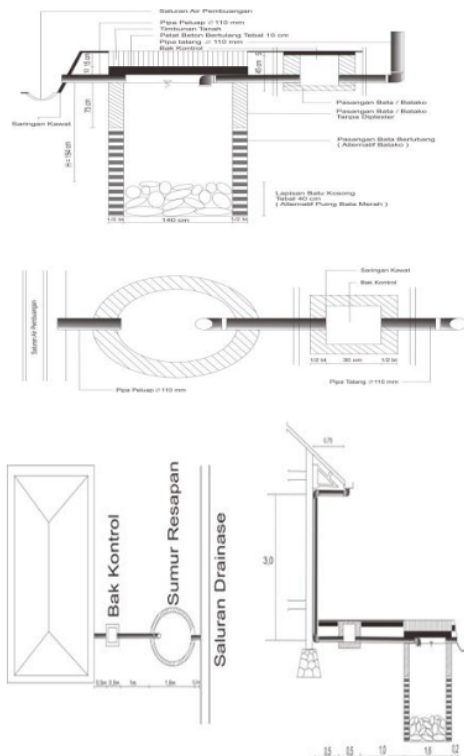
Gambar 6. Konstruksi Sumur Resapan
