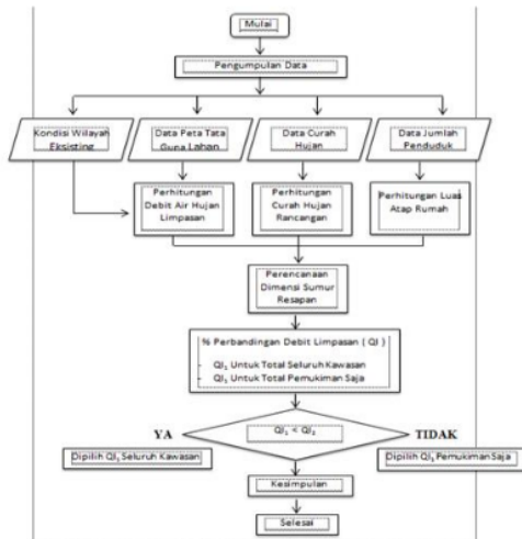
Gambar 5. Bagan Alir Kajian Sistem Drainase Sumur Resapan Air Hujan
