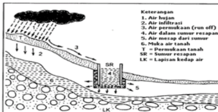
Gambar 3. Prinsip Kerja Sumur Resapan
