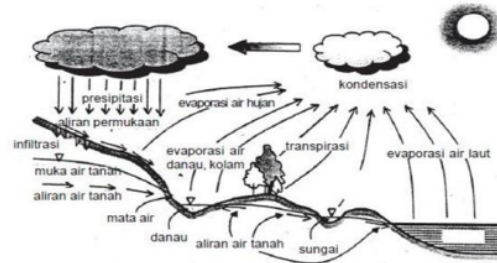
Gambar 1. Siklus Hidrologi
