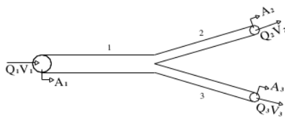
3 Gambar 2.4 Hukum Kontinuitas pada Pipa Bercabang
