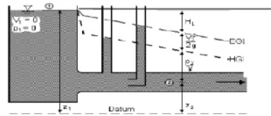
Gambar 2.2 Diagram Energi dan Garis Tekanan
