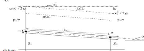
Gambar 2.1 Gradien Hidrolika
