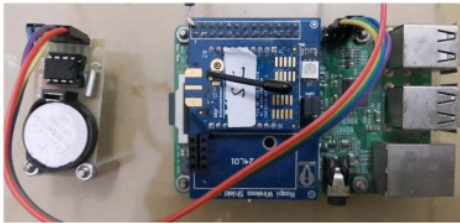
Fig. 2. Smart Controller module.
