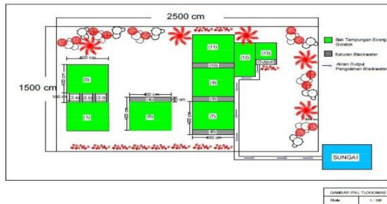
Gambar 8. Denah IPAL Komunal Tlogomas
