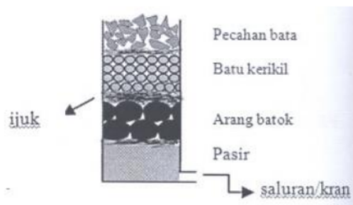
Gambar 6. Susunan material filter pada alat penjernih air sungai
