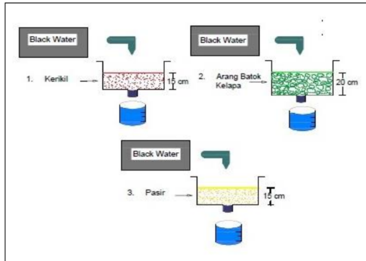
Gambar 7. Skema Pengolahan blackwater dengan filter tunggal
