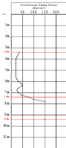
Gambar 6. qc1, qc2 dan JHP rata-rata pada Data Sondir
