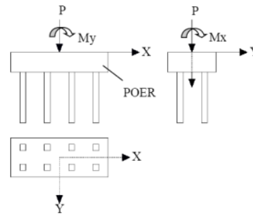
Gambar 1. Skema Pondasi Tiang Kelompok
