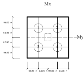
Gambar 9. Dimensi pilecap Pondasi Tipe 1
