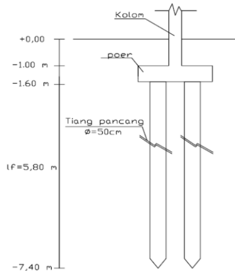
Gambar 5. Perencanaan Pondasi
