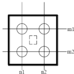
Gambar 8. Susunan Pondasi Tipe 1 (4 tiang)
