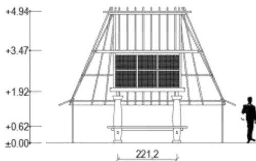
POTONGAN- A
