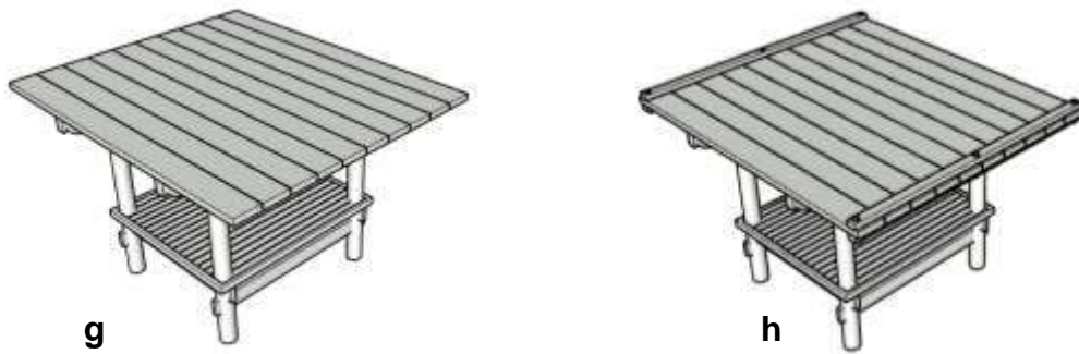
Gambar 3.87. (g) Yang dilakukan selanjutnya adalah memasang papan gelampar menumpu pada balok karang ulu . Ketebalan dari papan gelampar ini cukup tebal sehingga tidak melendut ketika menumpu di atas balok karang ulu . (h) agar papan gelampar stabil maka dikunci dengan cara digapit dengan dua balok di dua ujung papan, agar gepitan kuat maka diikat dengan pasak di tiga titik.
