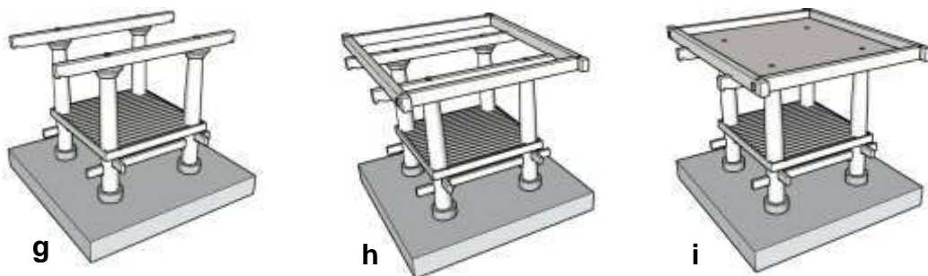
Gambar 3.24. (g) Pemasangan selanjutnya adalah memasang balok galang . (h) Kemudian dilanjutkan dengan memasang rangkaian balok blandar . (i) Dilanjutkan dengan pemasangan gelampar yaitu lantai tempat penyimpanan.
