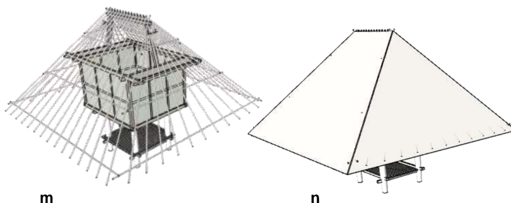
Gambar 3.41. (m) Semua kerangka sudah terpasang, untuk menahan panjangnya tritisan maka gepit bagian paling ujung bawah ditahan oleh batang bambu yang dikaitkan/ditumpangkan pada balok meret/blandar . (n) kemudian dilanjutkan dengan memasang bahan utama atap yaitu rangkaian ijuk yang diikatkan pada bilah bambu.
