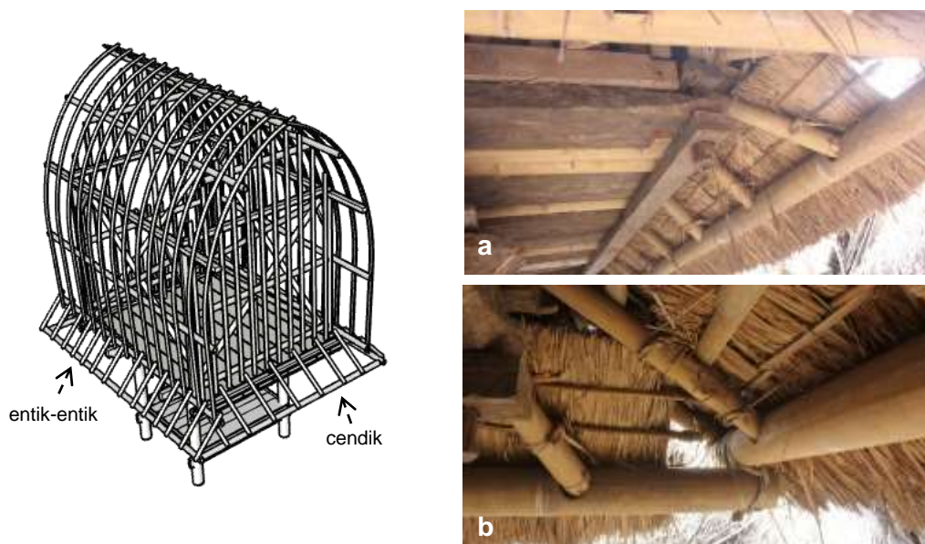
Gambar 4.50. Pemasangan cendik dan entik-entik (a) ujung bawah cendik diikat gapit . (b) gapit entik-entik menumpang pada gapit cendik (gambar dan photo : Gatot AS)
