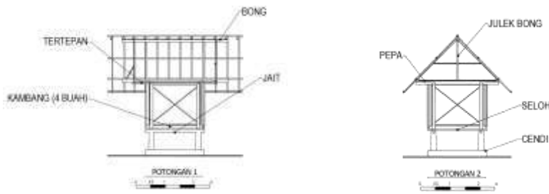
Gambar 3.55. Nama-nama istilah yang ada pada Sambu Gumantar . Ada beberapa istilah yang tidak tercantum, adalah: sapak sambu adalah papan lantai sambu ; anak dara adalah papan lubang pembuangan pada saat membersihkan sambu (berada di tengah-tengah sapak ).
