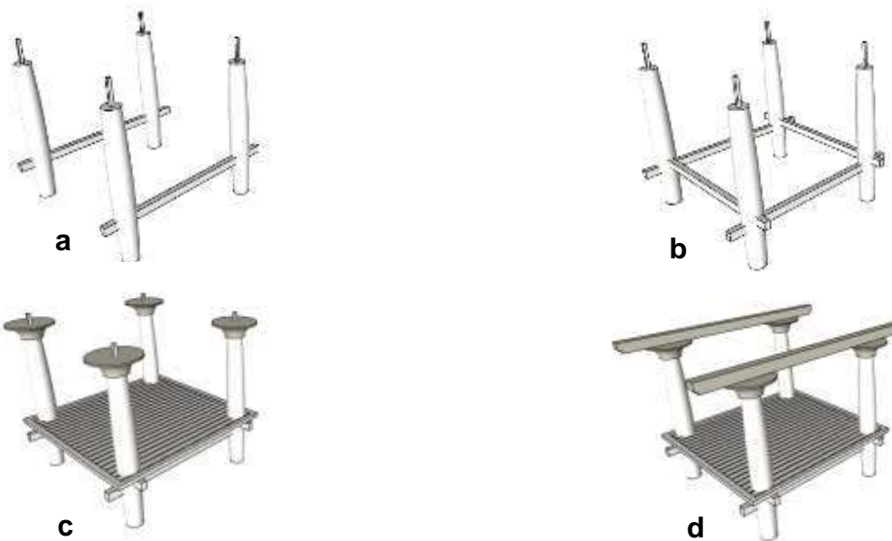
Gambar 3.36. (a) Pertama kali yang dirangkai adalah empat tiang dirangkai menjadi dua pasang dirangkai dengan jiat pendek . (b) Kemudian dua pasang tiang dirangkai menjadi satu dengan jiat tinggi , dengan cara memasukkan batangnya pada lubang yang telah ada di tiang. (c) Setelah terangkai keempat tiang baru diletakkan di atas cendi yang sudah disiapkan sebelumnya. Kemudian dilanjutkan dengan memasang aton (rangkain balok kayu sebagai pengunci bagian bawah yang bisa digunakan untuk tempat duduk). kemudian baru dipasang jelepeng . (d) Langkah selanjutnya adalah memasang balok penyangga dengan diletakkan di atas jelepeng .
