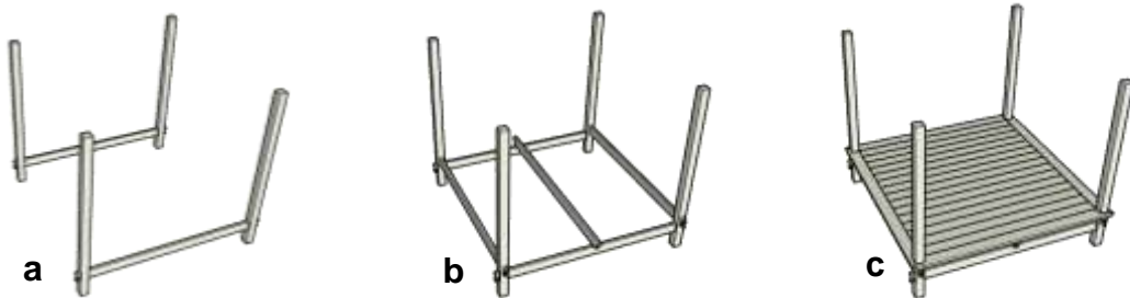
Gambar 3.81. (a) Pertama kali yang dirangkai adalah empat tekan (tiang), dijadikan dua pasang diikat dengan balok seloh . (b) Beru kemudian dipasang balok selanjutnya yaitu balok gegolok terletak dibagian tengah menumpu di seloh , dan dua balok jait masuk kelubang purusan di tekan . (c) Baru kemudian dipasang perangkat amben yaitu balok baton dan pengeret sebagai pengunci baru kemudian di kasih papan sebagai alas berugaq yang numpu di balok jais dan gegolok .
