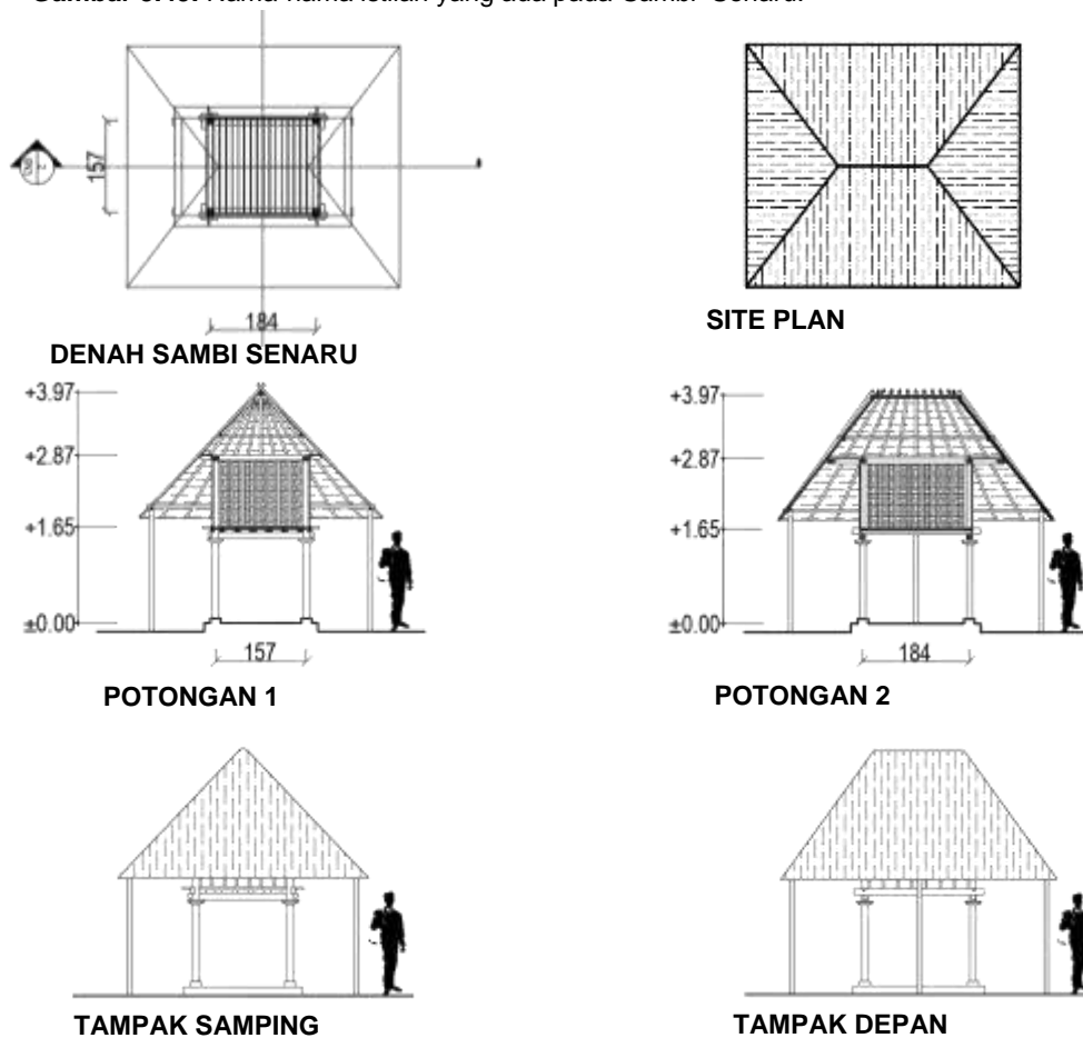
Gambar 3.49. Nama-nama istilah yang ada pada Sambu Senaru.
