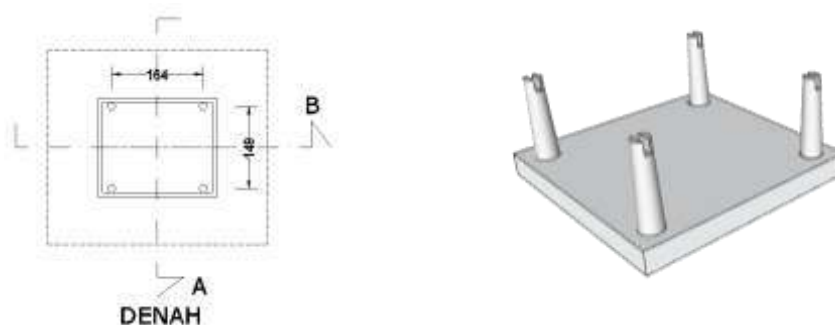
Gambar 4.22. pemasangan tiang Sambu (gambar: Gatot AS)
