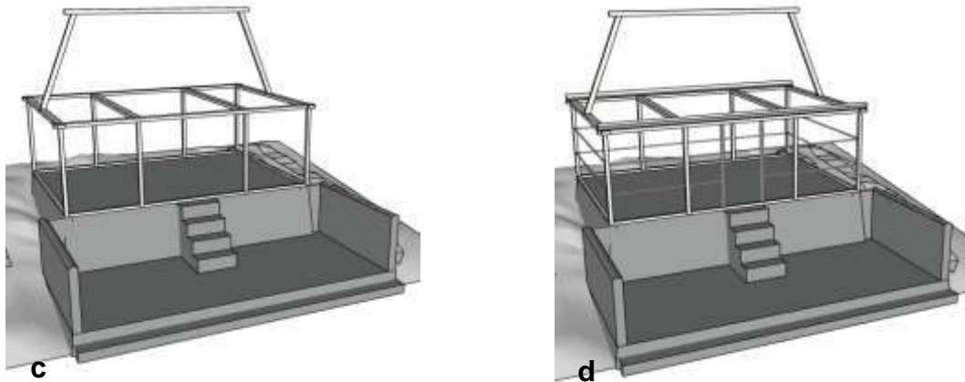
Gambar 3.4. (c) setelah rangka dinding terpasang, maka rangkaian pendukung atapnya ( panjang dan otak ) dirangkai numpu di lempen . Untuk menahan agar bisa berdiri maka dikanan kirinya ditahan batang bambu. (d) Kemudian balok kayu memanjang ( belandar ) dipasang menumpu di atas lempen . Demikian juga dengan kerangka dindingnya juga dipasang.
