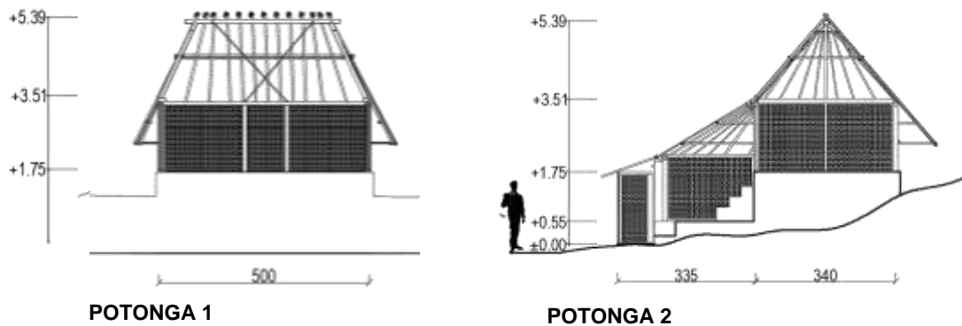
Gambar 3.74. Gambar Bale Tani rumah adat Sade.
