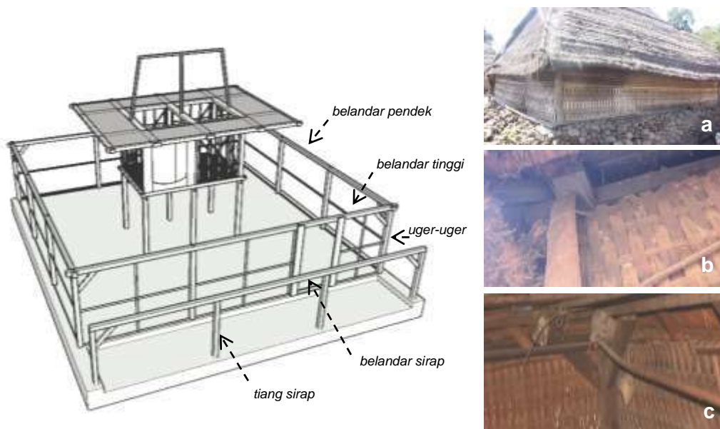
Gambar 4.82. Kerangka dinding pembatas (a) dinding pembatas menggunakan anyaman bambu, (b) pertemuan di sudut di ' tlangkup ' dengan batang bambu, (c) sistem struktur penyiku (gambar dan photo: Gatot AS).
