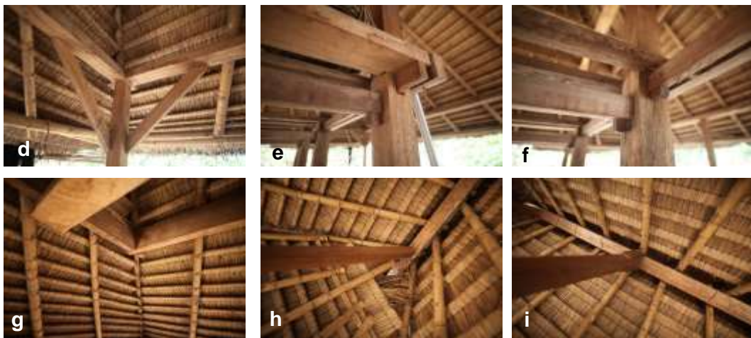
Gambar 2.42. Kode sampel BG 3 adalah Bale Mengina milik Rumansim di desa Beleq Gumantar. (a dan b) Tampak dari Bale Mengina, yang masih dalam tahap penyelesaian (c) Suasana ruang dalam, terlihat perangkaian struktur utama Bale Mengina. (d) Nampak sambungan pada bagian sudut luar. (e dan f) Rangkaian balok pada inaq bale, di sini terlihat bahwa inaq bale dan kakinya tidak terpisah, tiangnya menjulang sampai atas. (g) Rangkaian pada bagian sudut atas inaq bale. (h) pendukung nok pada bagian samping. (i) pendukung nok pada bagian tengah. (photo: Gatot A S)
