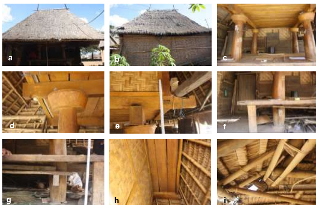
Gambar 2.10. Kode sampel LBB 4 adalah Panteq milik A Ratisah di Limbungan Barat, (a dan b) tampak Panteq , seperti halnya Panteq LBB 2 salah satu sisi ditutup. (c) Suasana ruang duduk yang sejuk. (d) Jelepeng adalah bentuk bulat di atas tiang sebagai pembatas antara ruang penyimpanan padi dan ruang duduk, (e) Rangkaian balok kayu yang menopang tempat penyimpanan padi. (f dan g) Rangkaian balok penompang bagian tempat duduk. (h) bagian tempat memasukkan padi. (i) pada bagian ujung atap tidak langsung lurus dari atas, namun dibelokkan lebih datar. (photo: Gatot A S)
