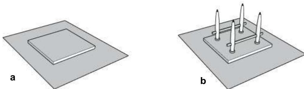
Gambar 3.10. (a) Pertama kali yang disiapkan adalah tempat berdirinya tiang Panteq di atas cendi . Dimana sebelum tiangnya ditumpukan permukaan cendi ditutup dengan ijuk. (b) Kemudian sepasang tiang didirikan, dimana tiap pasang tiang diikat dengan balok kayu dibagian bawah ( jait kontek ).
