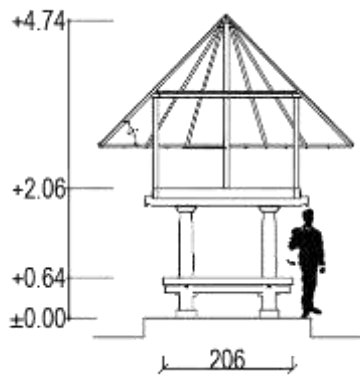
POTONGAN A
