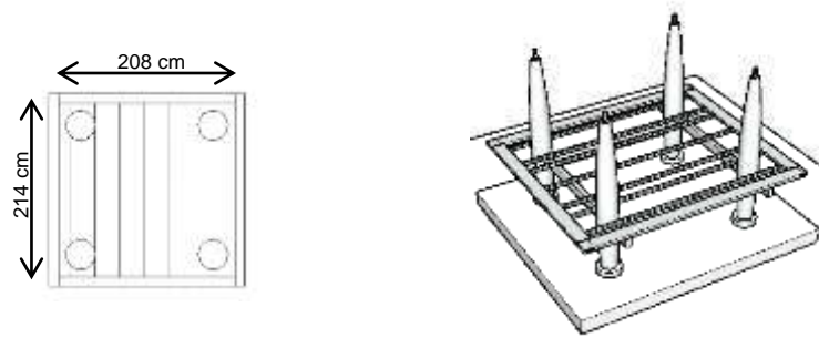
Gambar 4.42. perangkaian kerangka amben (gambar: Gatot AS)
