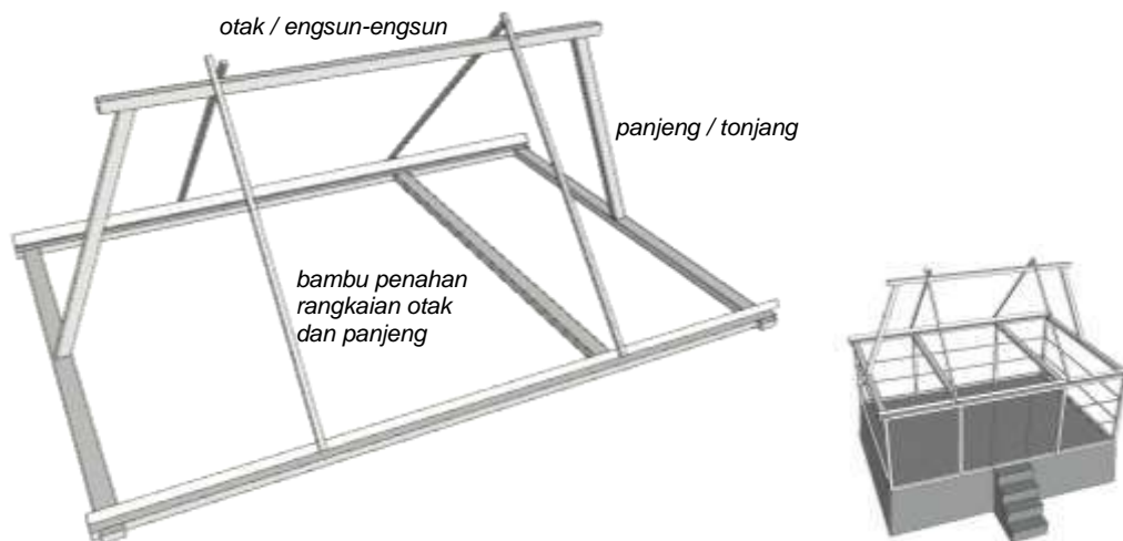
Gambar 4.7. Rangkaian balok panjang dengan balok otak di Bale Tani (gambar: Gatot AS)
