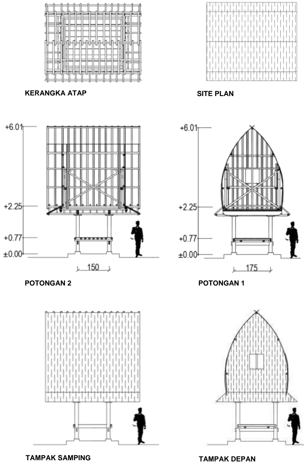
Gambar 3.85. Gambar Bale Alang rumah adat Sade.
