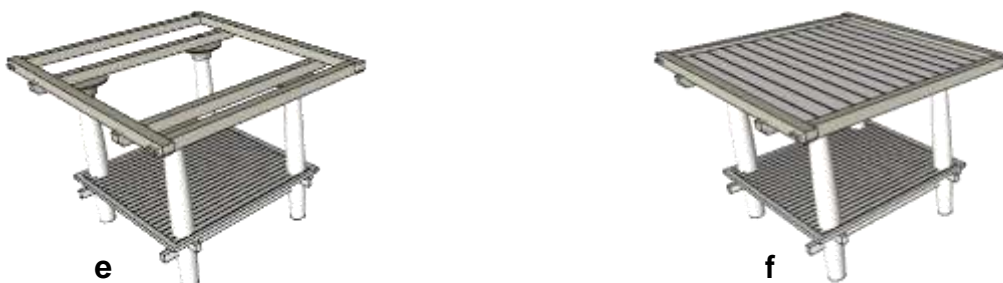
Gambar 3.37. (e) Setelah balok penyangga siap kemudian dilanjutkan dengan memasang balok penggeret yang merupakan rangkain balok kayu sebagai tumpuan bawah tempat penyimpanan. (f) Kemudian baru papan gelamparnya dipasang.
