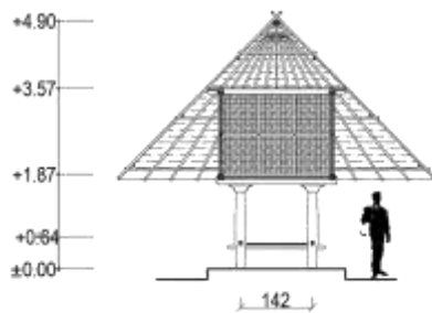
POTONGAN 1
