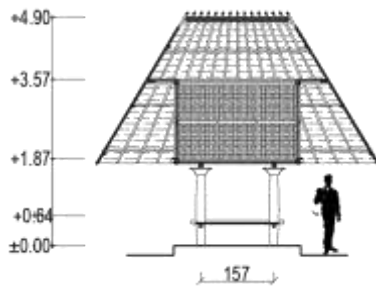
POTONGAN 2
