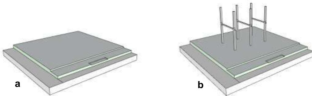
Gambar 3.62. (a) Terlebih dahulu lahan tempat berdirinya Bale Mengina dipersiapkan. (b) Kemudian keenam tiang dirangkai menjadi tiga pasang dengan menggunakan balok celoh dengan cara memasukkan bagian kedua ujungnya ke dalam lubang purusan di tiang. Baru kemudian diperkeras dengan menggunakan pasak.
