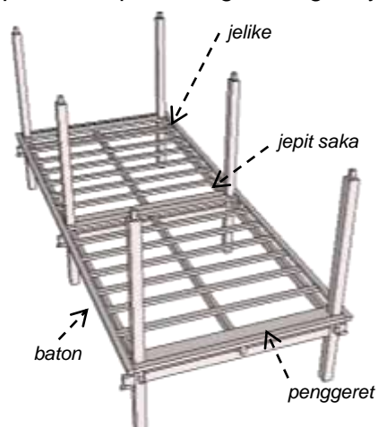
Gambar 4.67. Merangkai amben . (gambar dan photo: Gatot AS)
