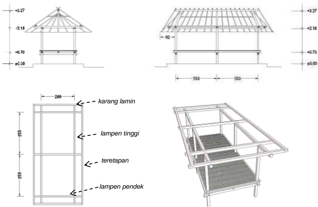
Gambar 4.69. Perangkaian struktur pendukung atap Berugaq . (gambar: Gatot AS)
