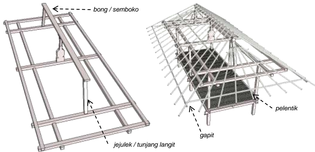
Gambar 4.71. Pemasangan kerangka atap Beruqaq . (gambar: Gatot AS)
