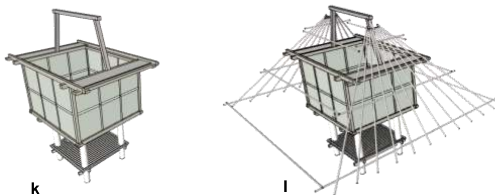
Gambar 3.40. (k) Kemudian dilanjutkan dengan pemasangan dinding penutup tempat penyimpanan yang bahan pokoknya menggunakan anyaman bambu. (l) Selanjutnya memasang kerangka atap, bisa dimulai dari bagian yang segitiga lebih dahulu dan baru kemudian bagian yang trapesium. Namun hal ini bisa urutannya dibalik dimulai dari yang trapesium terlebih dahulu. Peranan gapit ( bambu yang melintang di bawah kerangka atap) dalam perangkaian ini sangat penting karena berfungsi untuk membentuk dan meluruskan kerangka atap. Ikatan antara kerangka dan gapit dengan teknik ikatan.
