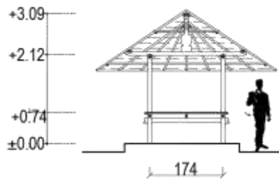
POTONGAN 1
