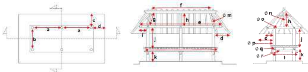
Gambar 4.62. Kitmap data sampel Berugaq (gambar: Gatot AS)
