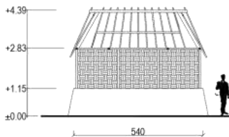
POTONGAN A
