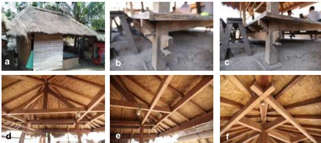
Gambar 2.60. Kode sampel SD 9 adalah Beruqaq milik Amaq Winah di Sade. (a) Tampak Beruqaq . (b dan c) Sistem sambungan balok pada bagian kaki, mirip dengan beruqaq Gumantar dan Senaru. (d, e, dan f) Sistem struktur bagian atas merupakan perpaduan sistem struktur lama dan sistem kuda-kuda baru. (photo: Gatot A S)
