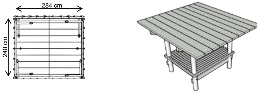
Gambar 4.46. memasang gelampar (gambar: Gatot AS)
