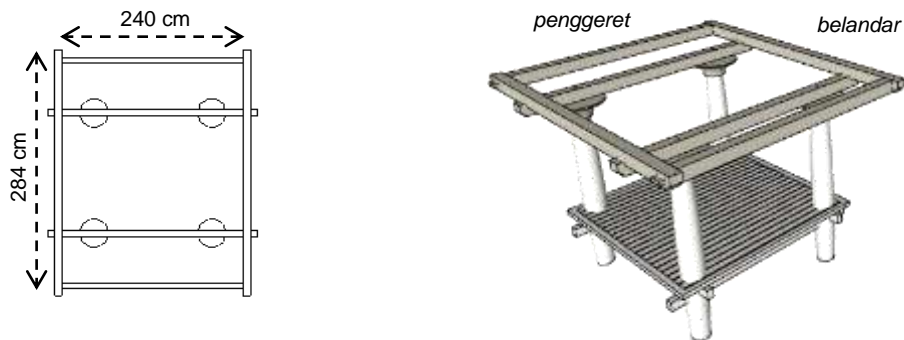
Gambar 4.51. merangkai balok belandar dan pengeret untuk tipe Geleng (gambar: Gatot AS)
