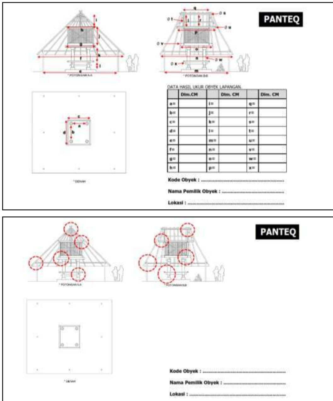
Gambar 1.14. Salah satu contoh format tabel pengambilan data dilapangan yaitu mengenai pengukuran dimensi gelagar dan pedoman pengamatan detail yang akan di diambil dengan sketsa atau photo.
