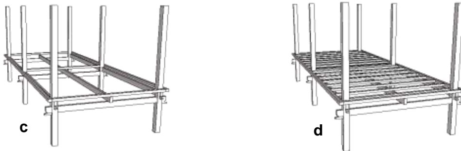
Gambar 3.45. (c) Kemudian memasang gegolok sebagai pengunci yang mengelilingi seluruh sakak . Tumpuan dari gegolok ini adalah numpang di atas balok jait tinggi , dan pertemuan sudut gegolok menggunakan sistem purus. (d) Kemudian di atas gegolok dipasang jeliar (sebagai tumpuan alas tempat duduk).
