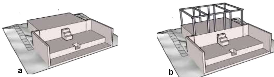
Gambar 3.75. (a) Pertamakali yang harus dilakukan adalah mempersiapkan lantena terlebih dahulu. Terdiri dari tiga tingkatan lante yaitu, bale dalam , sesangkok , dan orag-orag .(b) kemudian merangkai tiang teken dan lampen sebagai rangka dinding bale dalem . Sedangkan untuk dinding pembatas sesangkok menggunakan dinding dari tanah liat yang dicampur dengan kotoran sapi. Untuk dinding pembatas orag-orag yang samping merupakan kelanjutan dari dinding pembatas sesangkok , yang bagian depan menggunakan lembar rangkaian pintu, jendela dan pembatas (jawa: gebyok ).
