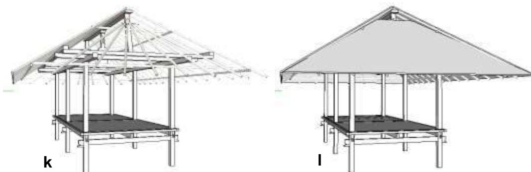
Gambar 3.48. (k) Adalah kerangka atap telah terpasang semua, sebagai catatan bahwa lembar atap yang berbentuk segitiga selalu di bawah dan yang berbentuk bujur sangkar atau yang memanjang di atasnya. Kalau ujung tritisan terlalu panjang maka biasanya bagian gapit terbawah disangga dengan tiang. (l) Atap dari bahan ilalang kemudian dipasang, dimulai dari bawah terlebih dahulu.
