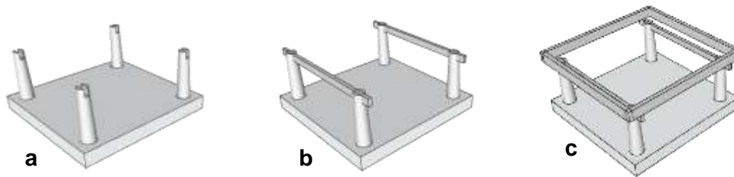
Gambar 3.57. (a) Pertama kali yang harus ditata adalah alas untuk berdirinya empat tiang yaitu cendi . (b) Kemudian empat tiang di ikat dengan jait menjadi dua bagian. (c) Kemudian di atasnya diberi rangkaian balok kambang yang terangkai berbentuk segi empat.
