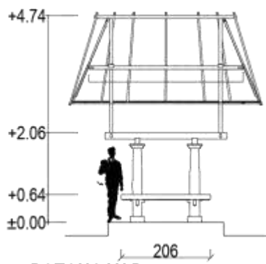
POTONGAN B
