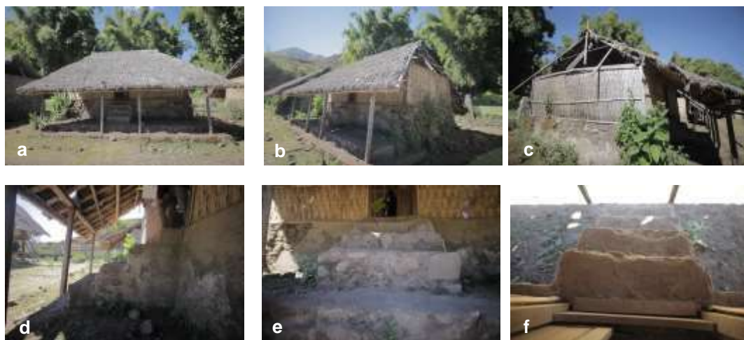
Gambar 2.16. Kode sampel SBL 1 adalah Bale-Tani milik Rumah Adat desa Beleq Sembalun. (a dan b) tampak Bale-Tani yang menunjukkan kondisinya yang sudah tidak dihuni lagi serta kondisinya yang rusak akibat gempa Lombok 2018. (c) Menunjukkan bahwa untuk menaikkan bangunan dengan menggunakan pasangan batu-kali, hal ini berbeda dengan yang ada di Limbungan. Apakah ini penyebab runtuhnya Bale-Tani di desa Beleq Sembalun ini? (d) 4 (empat) anak tangga digunakan pada Bale-Tani ini, nampak anak tangganya telah retak. Tangga terbuat dari susunan batu-kali, apakah hal ini yang menyebabkan retak terkena gempa Lombok 2018? (e sd g) Suasana ruang dalam Bale-Tani yang nampak rusak, terlihat di (e) penggunaan pintu geser untuk masuk ke ruang utama. Nampak juga di (g) adanya penyekatan ruang yang digunakan sebagai tempat orang tua, tempat melahirkan, dan tempat menazah. (h dan i) rangkaian struktur pendukung atap, penyangga tiang tegak kearah samping tidak ada, tegaknya karena adanya ikatan batang bambu pendukung atap. (j dan k) Beberapa penyelesaian sambungan antara bahan yang berbeda, bambu dan kayu. Pembuatan lubang pada batang kayu sebagai tempat menahan batang bambu yang dimasukkan di dalamnya. (l) Permainan estetika pada ujung tiang penyangga balok pada bagian depan. (photo: Gatot A S)
