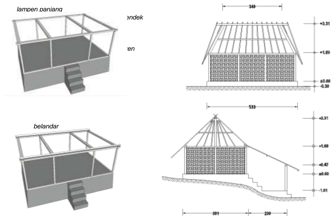
Gambar 4.5. Perangkaian struktur dinding pembatas inaq bale Bale Tani (gambar: Gatot AS)
