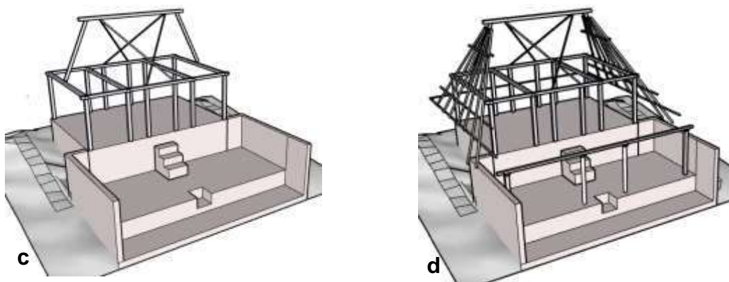
Gambar 3.76. (c) Setelah kerangka dinding bale dalem terangkai, dilanjutkan dengan merangkai balok tonjang dan ensun-ensun . Dua balok tonjang satu sisi menancap di atas balok lampen , dan sisi yang lain menopang balok ensun-ensun yang berfungsi sebagai balok bubungan. Agar tetap tegak rangkaian ini ditahan oleh balok bambu (seperti ikatan angin). (d) Sebelum pemasangan kerangka atap, maka terlebih dahulu dipasang balok belandar bale dalem dan belandar sesangkok . Belandar bale dalem numpang diatas balok lampen dan belandar sesangkok di tompang tiang.
