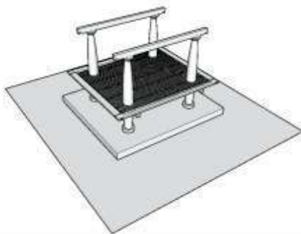
Gambar 4.45. posisi balok galang / penyangga / karang ulu menumpang di jelepeng (gambar/photo; Gatot AS)
