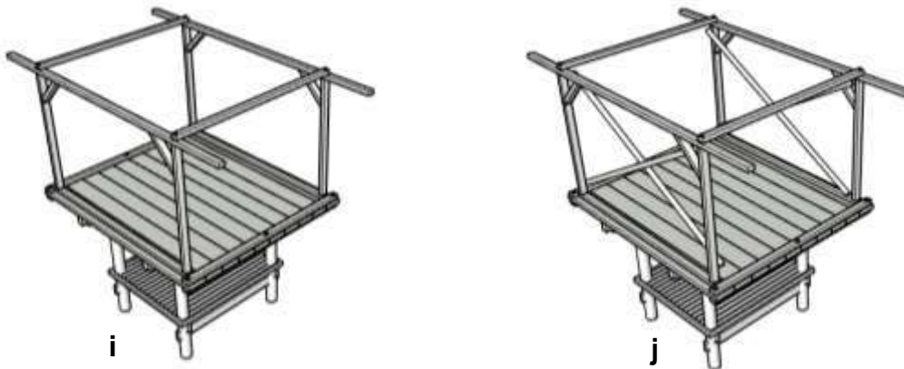
Gambar 3.88. (i) Setelah papan gelampar terpasang dan tidak goyang dilanjutkan dengan memasang kerangka ruang tempat penyimpanan. Keempat tiang ditancapkan masuk ke dalam papan gelampar , bagian ujung atas diikat dengan balok kayu dan diberi penyiku sehingga rangkaian ini tidak goyang. Kemudian kedua rangkaian tiang ini ditahan dengan dua balok melintang sehingga terbentuk kerangka ruangnya. (j) Supaya tidak goyang rangkaian ini diikat dengan kayu menyilang, sekaligus sebagai pegangan dalam perangkaian waras (kerangka atap bale alang ).
