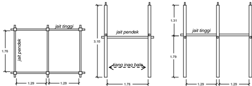
Gambar 4.76. Rangkaian tiang inaq bale (gambar: Gatot AS).
