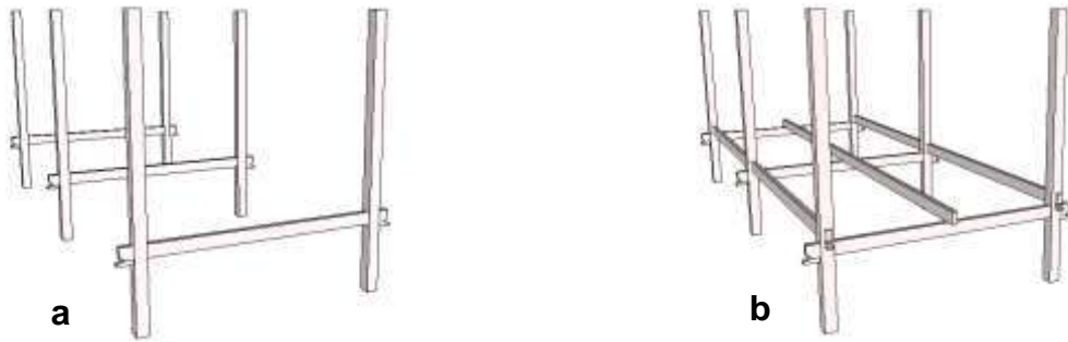
Gambar 3.44. (a) Yang pertama kali dirangkai adalah enam sakak dari berugaq, dijadikan tiga pasang rangkaian sakak. Adapun pengikat dua sakak dengan menggunakan balok jait pendek, yang dikerasi dengan menggunakan pasak. Berugaq dengan menggunakan enam sakak dinamakan sekenem. (b) Kemudian ketiga pasang sakak diikat jadi satu dengan menggunakan balok jait tinggi, dengan cara memasukkan jait tinggi pada lubang yang telah ada pada sakak. Posisi sakak sebelah tengah diatur supaya benar-benar ditengah, kemudian kalau sudah pas baru bikeri dengan menggunakan pasak.
