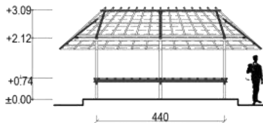
POTONGAN 2
