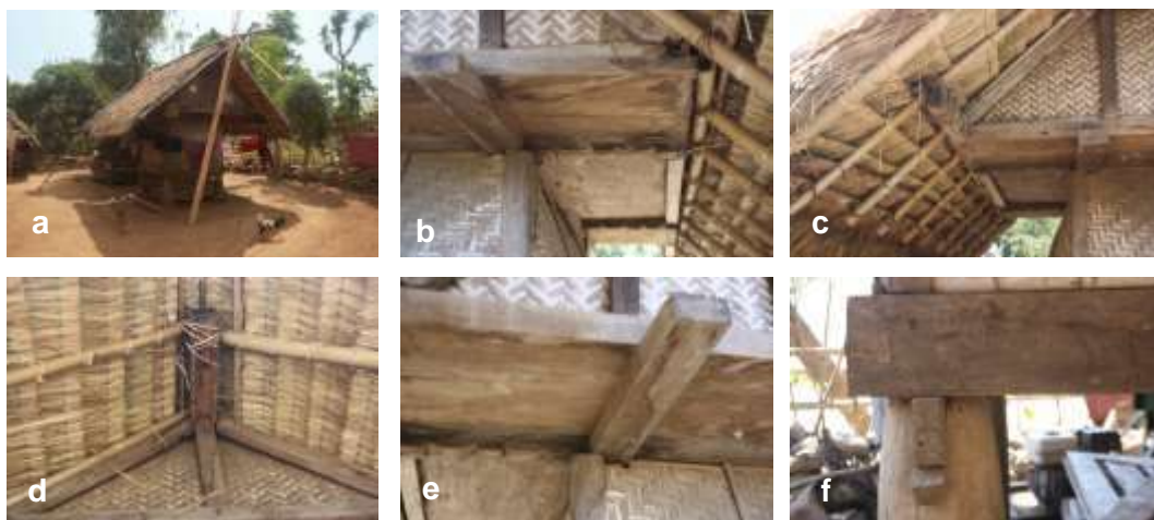
Gambar 2.39. Kode sampel BG 6 adalah Sambi milik Raden Ketanom di desa Beleq Gumantar. (a) Tampak Sambi , bentuknya mirip dengan Sambi yang lain. (b dan c) Rangkaian balok bagian atas tempat menyimpan padi. (d) Rangkaian balok tiang penyangga balok nok, yang menjadi satu dengan dinding pembatas tempat padi. (e) masih ada sedikit permainan estetika dengan mengukir batang kayunya. (f) Ada kemiripan sistem struktur pada bagian bawah Sambi ini dengan Sambi sebelumnya, BG 4 dan BG 5. (photo: Gatot A S)
