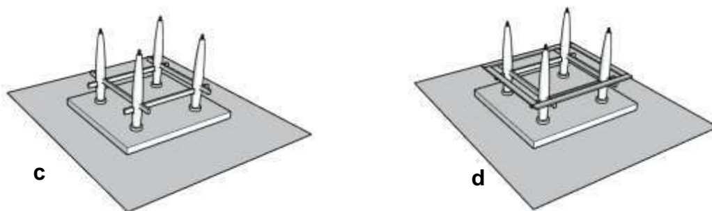
Gambar 3.11. (c) Agar tetap tegak keempat tiang, pasang dipasang balok melintang selanjutnya yaitu jait belo . Pada mulanya lubang untuk tempat masuknya jait belo ke tiang longgar, biar tidak longgar maka diganjal dengan pasak. Pada awalnya tidak terlalu rapat, perapatkan setelah rangkaian tiang ini selesai semua. (d) Selanjutnya pemasangan balok pengunci ( jelike ), sekaligus sebagai kerangka dari tempat duduk ( malak ) di atas ujung balok jait belo . Rangkai kerangka malak ini selain empat balok jelike yang mengelilingi malak , balok lain terpasang dibagian tengah menumpang pada balok jait belo ikut memperkuat malak . Posisi terpasangnya adalah seperti pada gambar 3.12.e. kemudian bisa juga dilanjutkan memasang bilah-bilah bambu yang di rangkai dengan rotan ( jejalin malak ), sehingga dapat dimanfaatkan sebagai injakan untuk pemasangan selanjutnya. Kalau sudah demikian maka rangkaian balok jait kontek dan jait belo pasaknya bisa diperkeras agar tidak terjadi goyangan. Di gambar 3.12.f. pemasangan bilah-bilah bambu malak dilakukan bersamaan dengan pemasangan galang (balok kayu membujur di atas jelepeng ), hal ini merupakan alternatif urutan lain yang dapat dilakukan.
