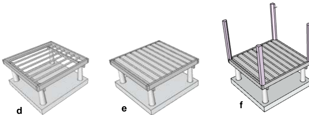
Gambar 3.58. (d) Setelah kambang dipasang, kemudian di dalamnya dipasang balok seloh yang menumpang di atas jait . (e) Kemudian dilanjutkan dengan memasang sapak sambu (papan lantai sambu). (f) Kemudian dipasang tiang yang posisinya di sudut kambang , dengan bentuk catokan yang khusus.
