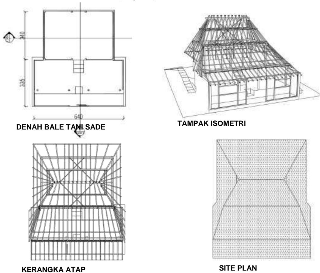
Gambar 3.73. Nama-nama istilah yang ada pada Bale Tani Sade .
