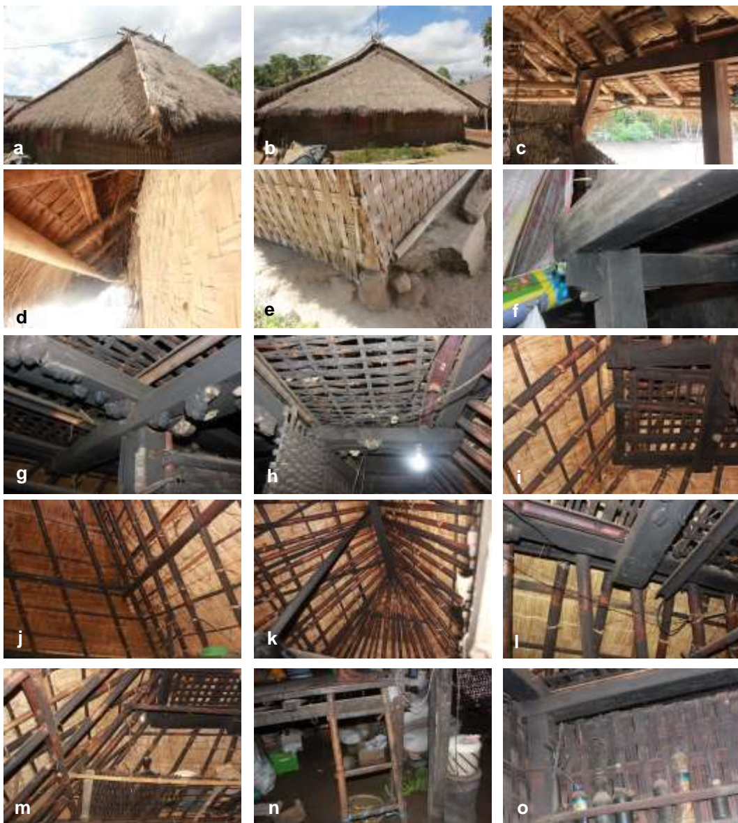
Gambar 2.22. Kode sampel SN 1 adalah Bale-Mengina milik Aldo di Senaru. (a, dan b) Tampak dari Bale-Mengina dan lingkungannya. (c) Penyelesaian sambungan balok arah horisontal dan vertikal dengan penyiku. (d) Sambungan balok pertemuan menyiku dibagian sudut depan. (e dan f) Sambungan di inaq bale menggunakan sistem pasak. (g) Menunjukkan pemasangan dinding inaq-bale, dipasang setelah rangka inaq-bale terpaasang terlebih dahulu. Menunjukkan bahwa dinding penyekat adalah bagian terpisah. (h) Penyelesaian sambungan kerangka atap ujung yang berbentuk segitiga. (g) Pengangga atap utama yang terletak dibagian tengah. (photo: Gatot A S)
