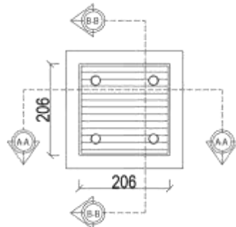
DENAH GELENG SEMBALUN
