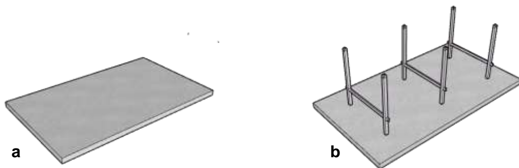
Gambar 3.69. (a) Sebagai tempat peletakan berugaq biasanya tanahnya dibuat lebih tinggi dibandingkan dengan sekitarnya, lalu disiapkan cendinya sebagai tempat tumpuan enam tiang berugaq . (b) Kemudian keenam tiang dirangkai menjadi tiga pasang dengan balok seloh dengan cara memasukkan ke dalam lubang tiang yang telah disiapkan, lalu diperkeras dengan menggunakan pasak.
