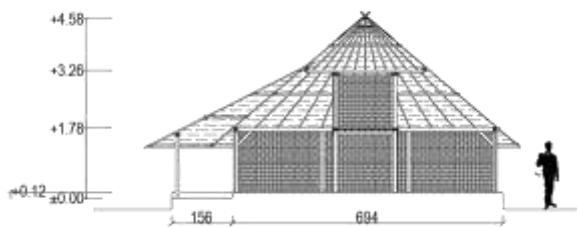
POTONGAN 1
