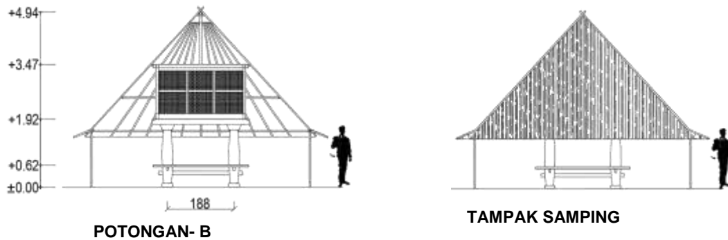
Gambar 3.9. Gambar Panteq Limbungan.
