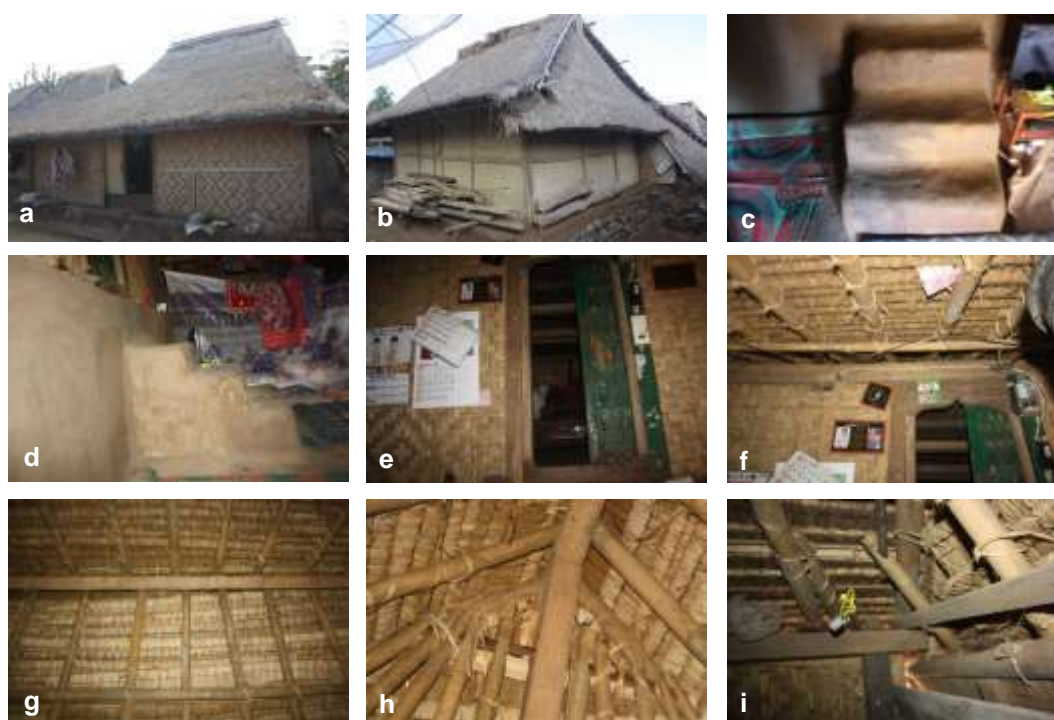
Gambar 2.5. Kode sampel LBT 1 adalah Bale-Tani milik Amaq Alfiah di Limbungan Timur, (a) adalah tampak depan Bale-Tani . (b) Tampak belakang Bale-Tani , bila dilihat dari tampak depan dan belakang tidak nampak konturnya. (c dan d) 3 (tiga) anak tangga menghubungkan ruang utama dengan ruang depan, ini menunjukkan masih adanya leveling walaupun tidak setinggi Bale-Tani sebelumnya. (e dan f) Memperlihatkan pintu masuk ke ruang utama dengan sedikit permainan estetika. (g, h, dan i) Struktur penyangga atap menggunakan bambu, dan struktur utamanya menggunakan balok kayu, (h) Terlihat penyelesaian khusus pada bagian atap segitiga, bagaimana merangkai kayu menjadi satu pada bagian atas. (photo: Gatot A S)
