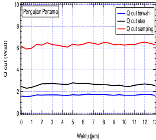
Gambar 3. Grafik Q out vs Waktu
