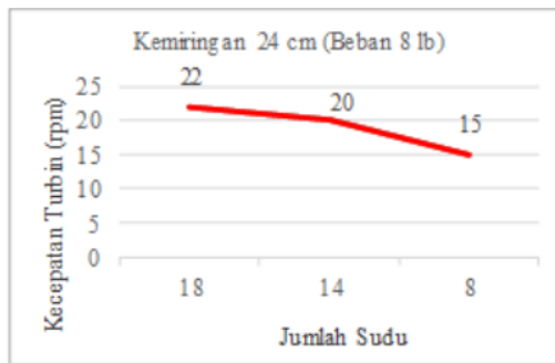
Gambar 1. Grafik jumlah sudu vs kecepatan turbin menggunakan kemiringan 24 cm dengan beban 8 lb.
