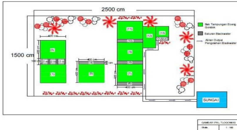
Gambar 1. Denah IPAL Komunal Tlogomas
