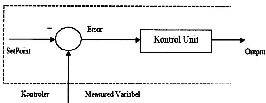
Gambar 3.10 Kontroler Dan Diagram Kotaknya
