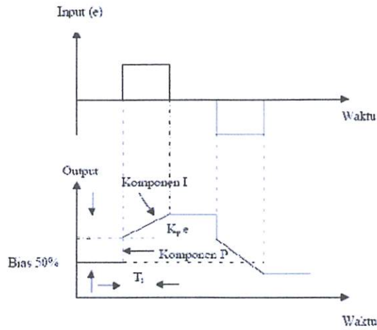
Gambar 3.15 Hubungan Input-Output Pengendali PI dalam Fungsi Waktu
