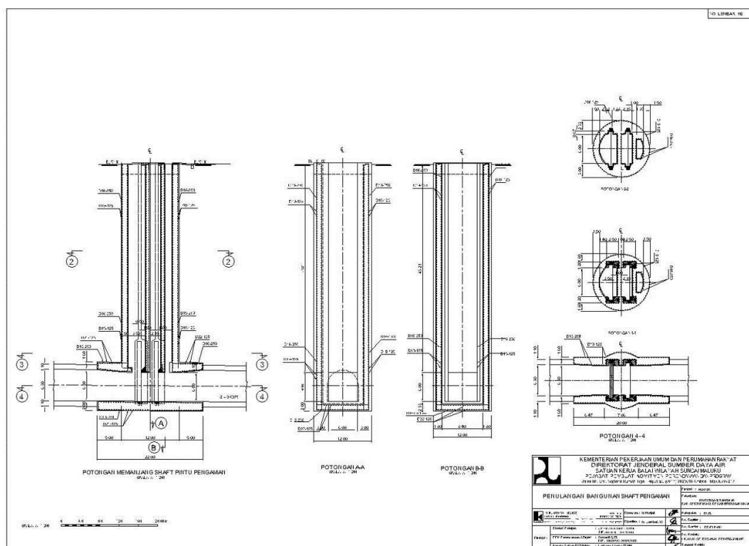
Lampiran 5 Penulangan Bangunan Shaft (sumber : PT.Indrakarya, 2017)
