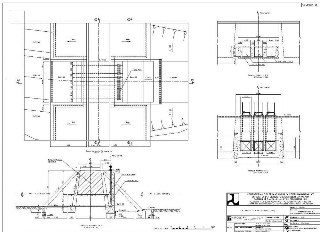
Lampiran 7 Konstruksi inlet Terowongan sumber : (PT.Indrakarya, 2017)
