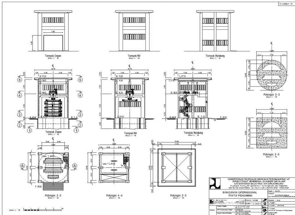
Lampiran 8 Bangunan Operasional Pintu Pengaman (sumber : PT.Indrakarya, 2017)
