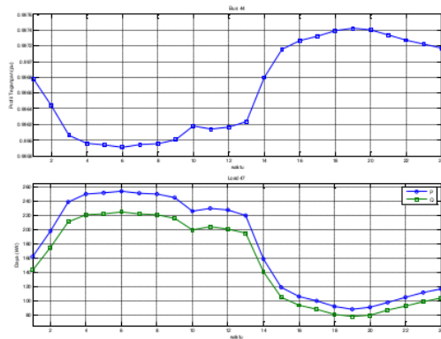
Gambar48. Gambar profil tegangan pada bus 44 dari penyulang Zaenal Zakse dan perbandingan profil tegangan dengan profil beban.
