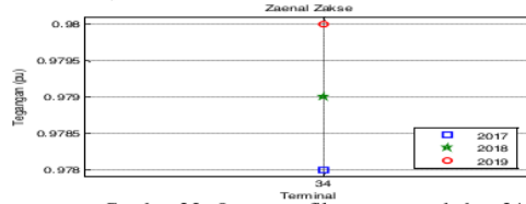
Gambar 32. Output profil tegangan pada bus 34 bus 36 = 0,98 PU
