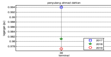
Gambar 15. Output profil tegangan pada bus 39 bus 55 = 0,978 PU
