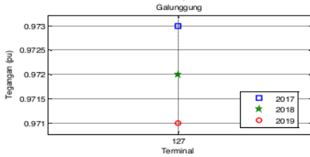
Gambar 22. Output profil tegangan pada bus 127
