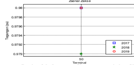
Gambar 36. Output profil tegangan pada bus 50 bus 52 = 0,977 PU
