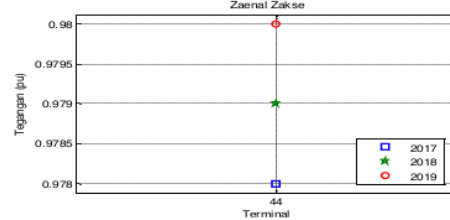
Gambar 35. Output profil tegangan pada bus 44 bus 50 = 0,98 PU
