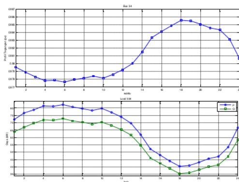
Gambar39. Gambar profil tegangan pada bus 34 dari penyulang Galunggung dan perbandingan profil tegangan dengan profil beban
