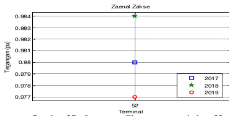
Gambar 37. Output profil tegangan pada bus 52
