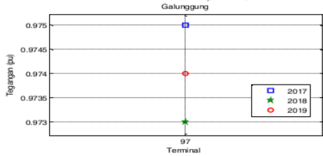
Gambar 20. Output profil tegangan pada bus 97 bus 103 = 0,975 PU
