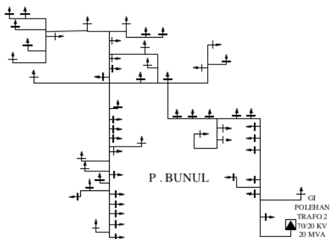
Gambar. 4. Single Line Diagram Feeder Bunul 20/0,4 kV
