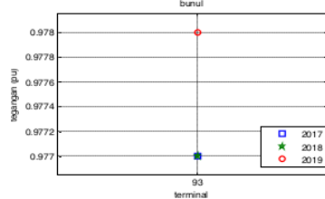
Gambar 30. Output profil tegangan pada bus 93
