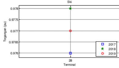
Gambar 26. Output profil tegangan pada bus 28 bus 53 = 0,979 PU
