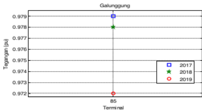
Gambar 19. Output profil tegangan pada bus 85 bus 97 = 0,973 PU
