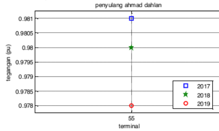
Gambar 16. Output profil tegangan pada bus 55
