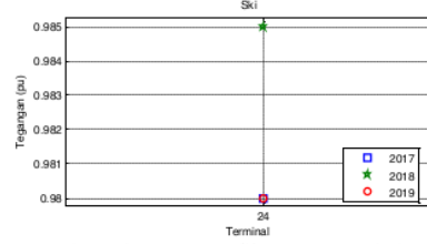
Gambar 25. Output profil tegangan pada bus 24 bus 28 = 0,978 PU
