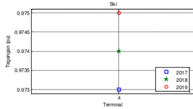
Gambar 24. Output profil tegangan pada bus 4 bus 24 = 0,985 PU
