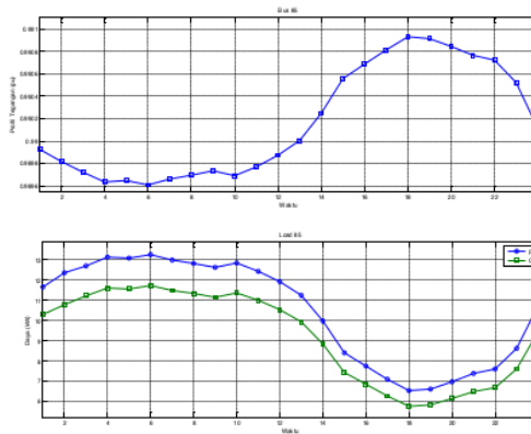
Gambar40. Gambar profil tegangan pada bus 85 dari penyulang Galunggung dan perbandingan profil tegangan dengan profil beban
