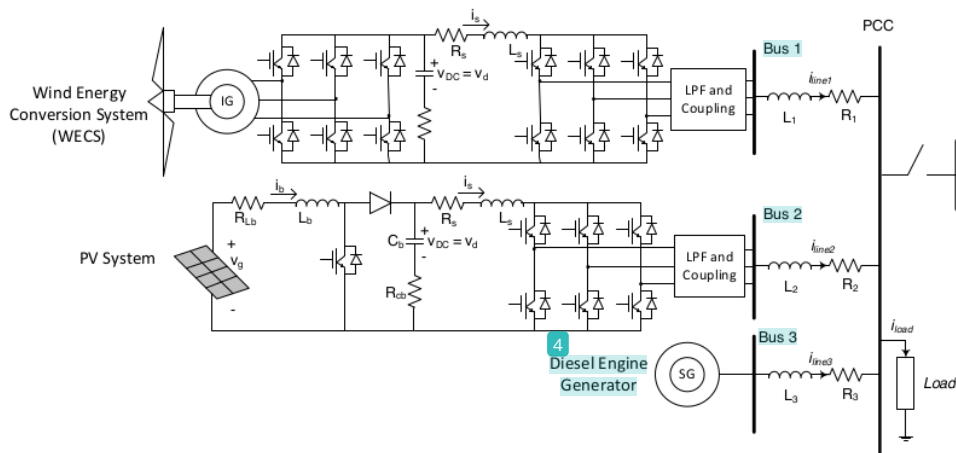
Gambar 2.3 Sistem Microgrid.
