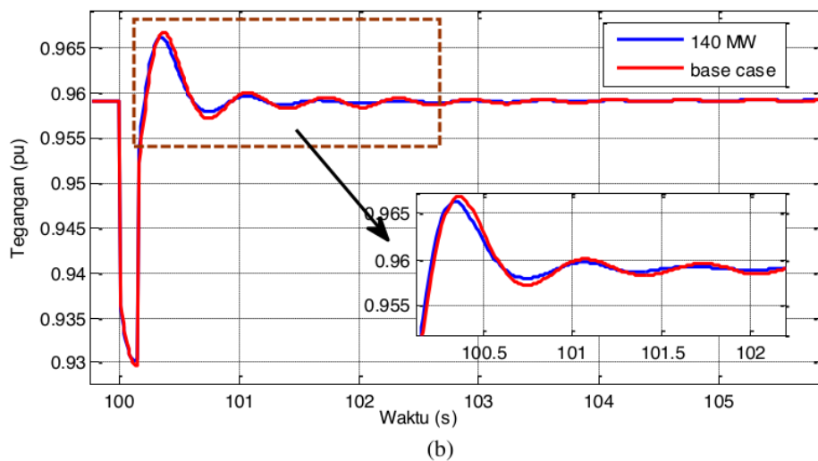
Gambar 4.4. Grafik Respon Tegangan Dinamik pada Bus (a) 30 dan (b) 31 ketika terjadi gangguan hubung singkat
