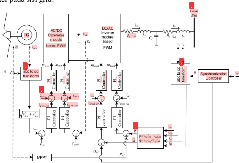
Gambar 2. Model Dinamik dari PLTB berbasis FRC.
