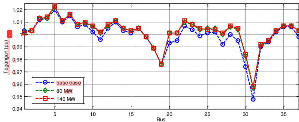
Gambar 4.2. Profil Tegangan Sebelum dan Sesudah Integrasi PLTB
