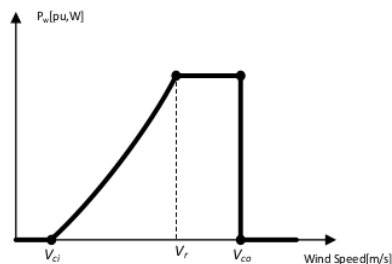
Gambar 1. Kurva Karakteristik Turbine Angin.
