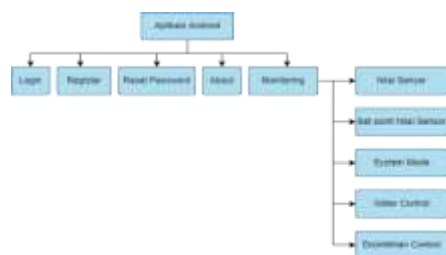
Gambar 3.2 Struktur Menu
