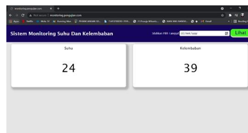
Gambar 10. Halaman Web
