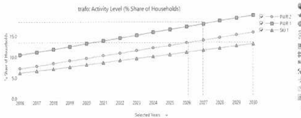
Grafik 4.1 Hasil simulasi LEAP daya beban trafo GI Sukorejo Purwosari tahun 2016-2030
