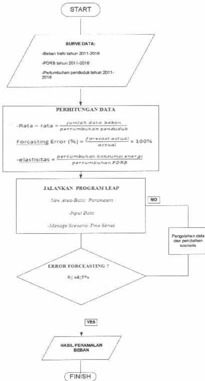
Gambar 3.2 Flowchart prakiraan beban listrik jangka panjang
