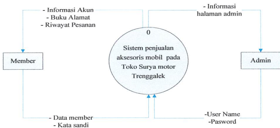
Gambar 3.2 DFD Level 0
