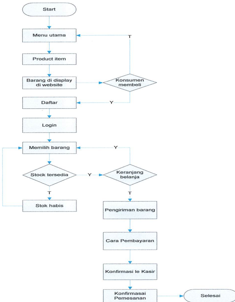
Gambar 3.1 Flowchart pembelian
