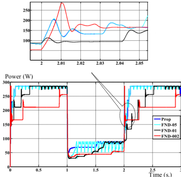
Gambar 2 Hasil Pengujian Teknik MPPT dengan Modifikasi Step Size
