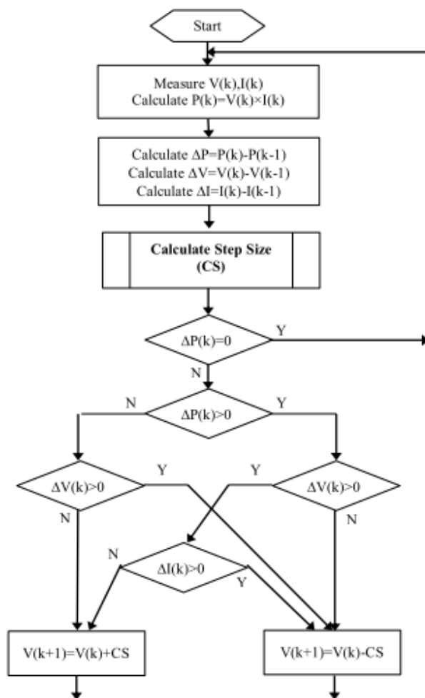
Gambar 1. Diagram alir teknik MPPT yang diusulkan peneliti [3]
