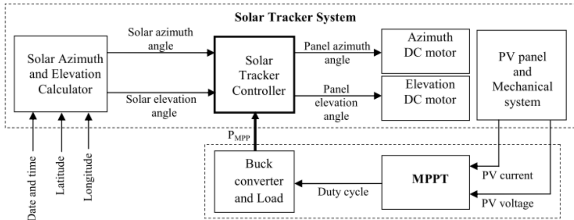
Gambar 3. Arsitektur Integrasi Solar Tracker dan MPPT [5]
