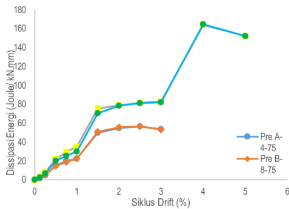
Gambar 6. Dissipasi energy benda uji
