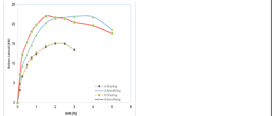
Gambar 3. Kurva Envelop Kapasitas Lateral
