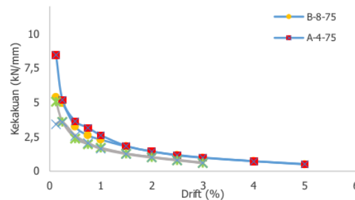
Gambar 5. Degradasi kekakuan
