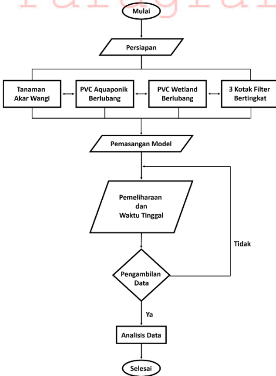
Gambar 6.1 Diagram alir eksperimen pengembangan IPAL
