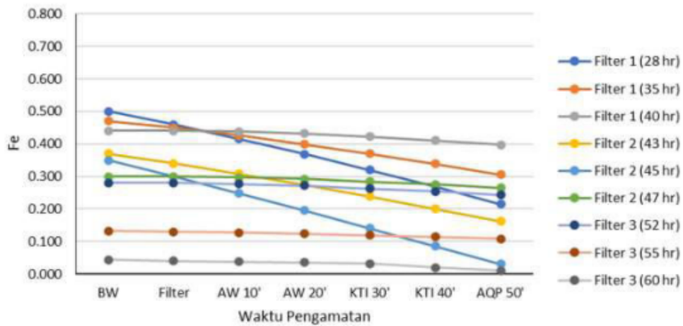
Gambar 7.14 Grafik penurunan kadar zat besi (Fe)
