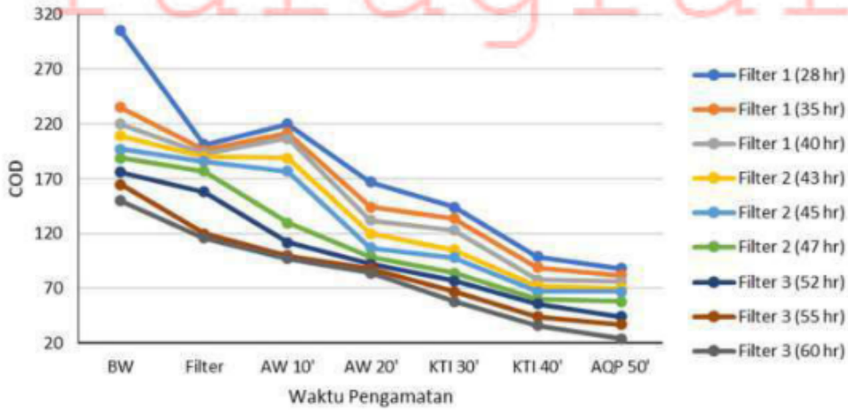
Gambar 7.11 Grafik penurunan kadar organik kimia (COD)
