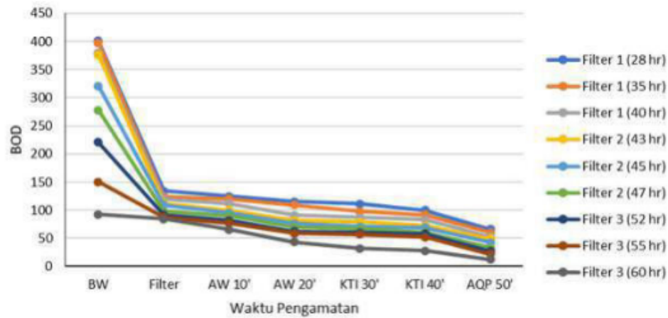
Gambar 7.8 Grafik penurunan kadar organik biologi (BOD)
