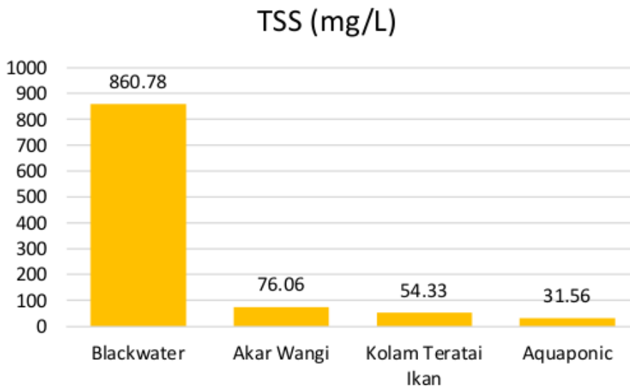
Gambar 7.1 Hasil pengukuran padatan tersuspensi (TSS)
