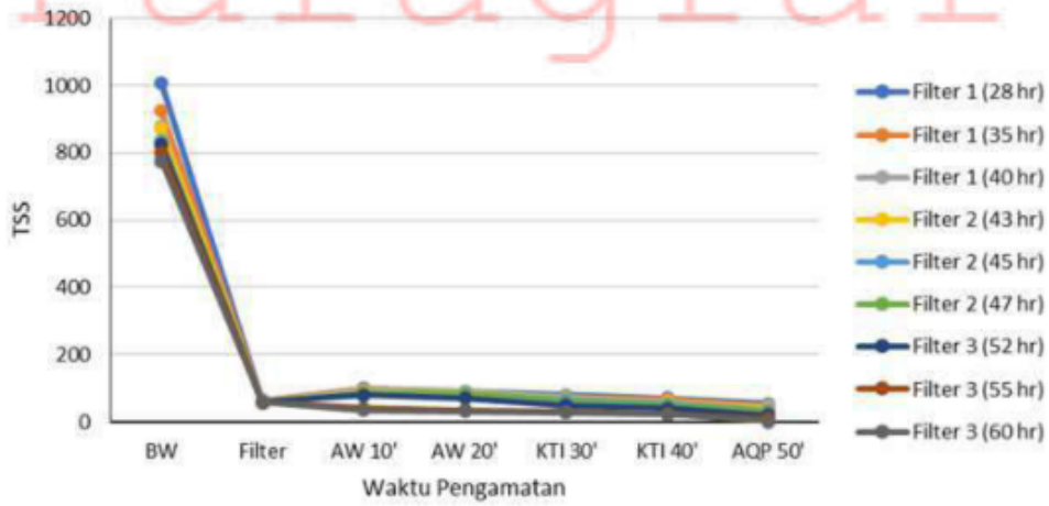
Gambar 7.2 Grafik penurunan kadar padatan tersuspensi (TSS)
