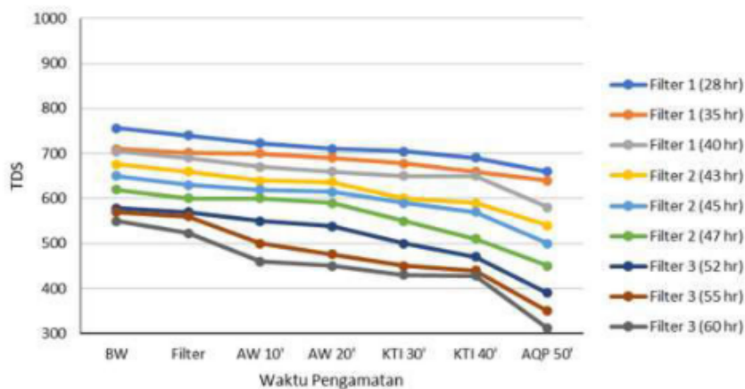
Gambar 7.5 Grafik penurunan kadar padatan terlarut (TDS)
