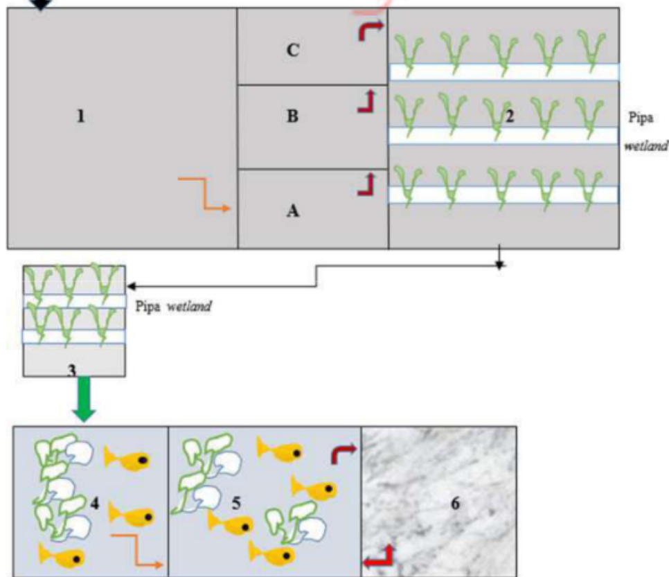
Gambar 6.2 Kosep pengembangan IPAL dengan penambahan tiga teknik yang dipadukan; filtrasi bertingkat (A,B,C), lahan basah buatan (2,3), serta akuaponik (4,5)
