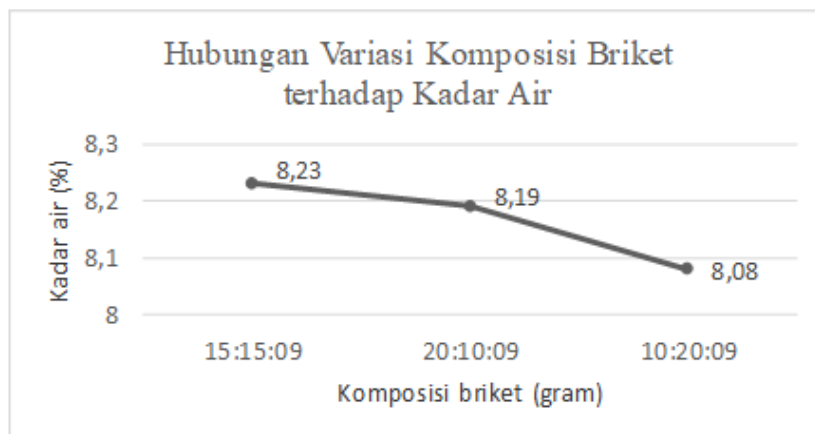
Gambar 2. Grafik pengaruh variasi komposisi briket terhadap kadar air
