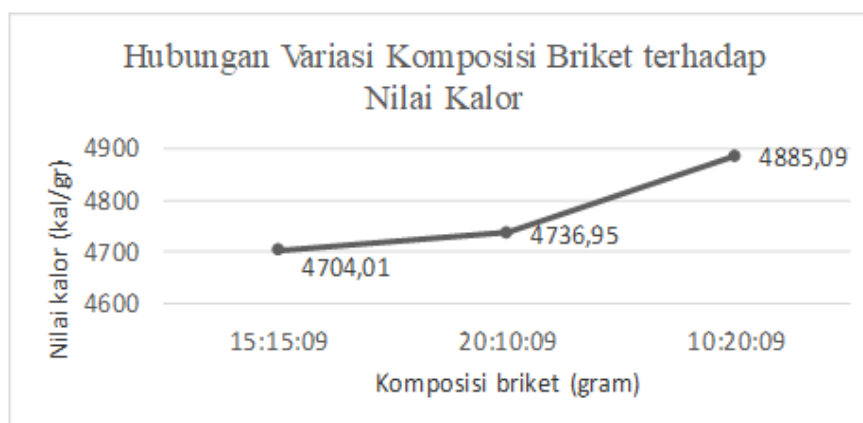
Gambar 1. Grafik Hubungan Variasi Komposisi Briket Terhadap Nilai Kalor
