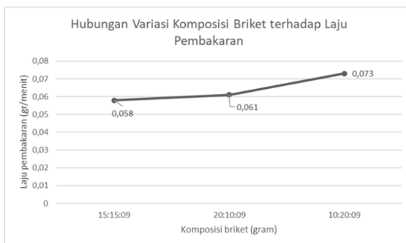
Gambar 3. Grafik hubungan variasi komposisi briket terhadap laju pembakaran
